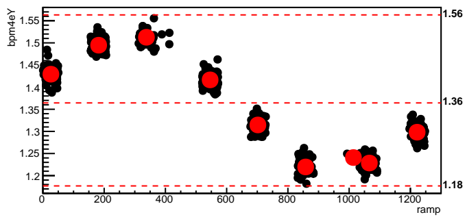
bmod_trim4,cyc=4895
