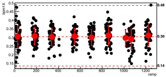
bmod_trim4,cyc=4895
