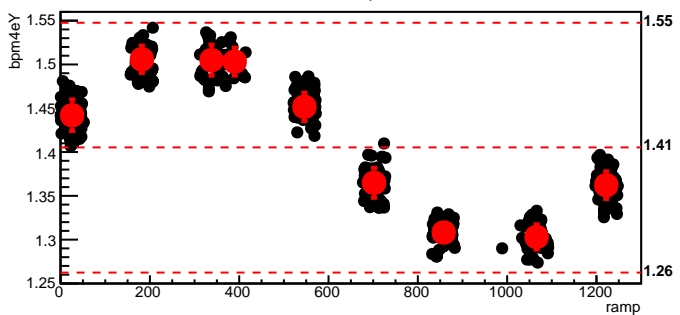
bmod_trim2,cyc=4895
