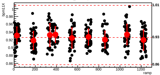
bmod_trim4,cyc=4911
