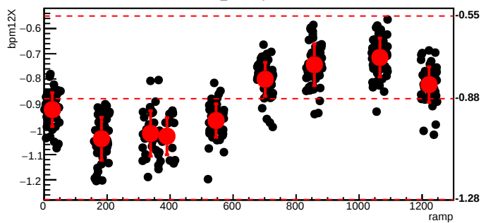
bmod_trim1,cyc=4911
