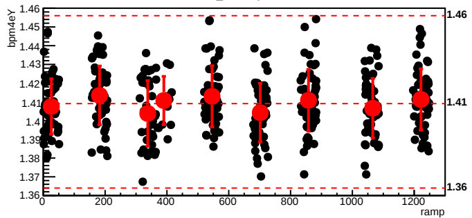
bmod_trim5,cyc=4911
