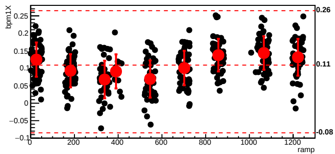
bmod_trim3,cyc=4911
