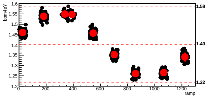
bmod_trim4,cyc=4911
