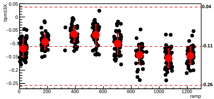
bmod_trim3,cyc=4951
