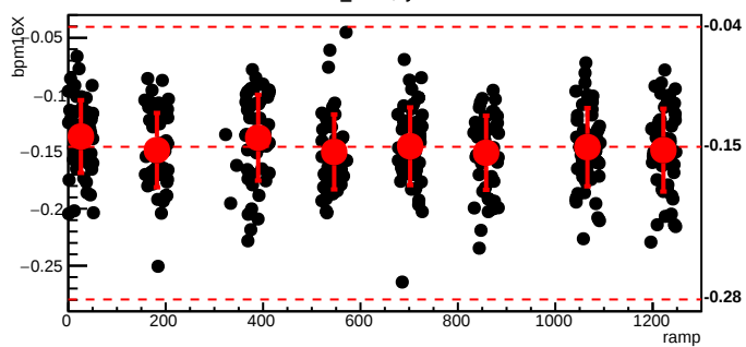
bmod_trim6,cyc=4951
