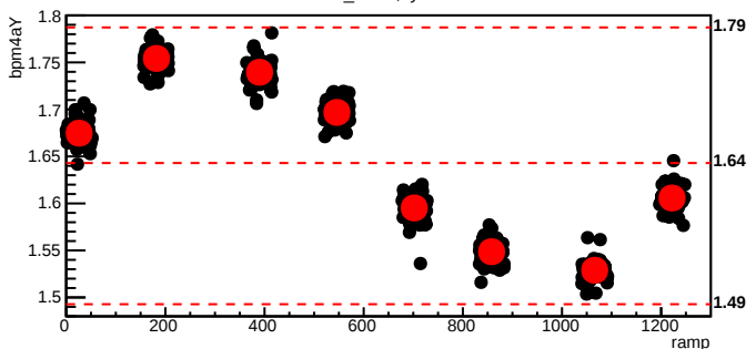
bmod_trim2,cyc=4951
