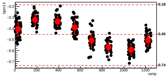
bmod_trim7,cyc=4951
