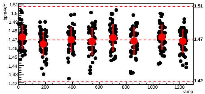
bmod_trim7,cyc=4951
