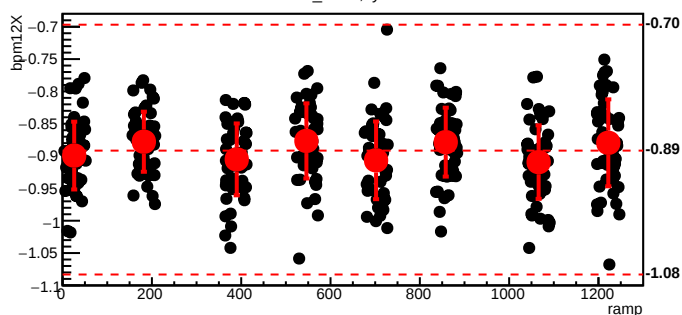
bmod_trim2,cyc=4951
