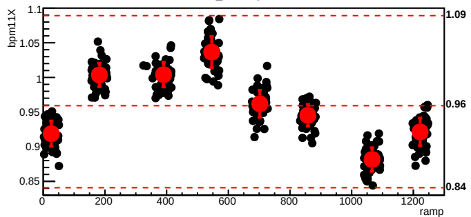
bmod_trim5,cyc=4951
