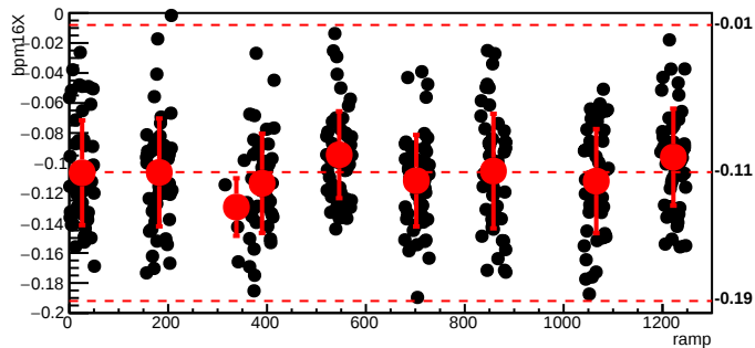
bmod_trim4,cyc=4951
