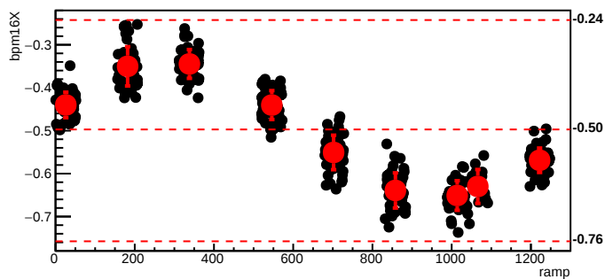
bmod_trim1,cyc=5167
