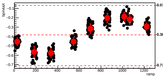
bmod_trim1,cyc=5167
