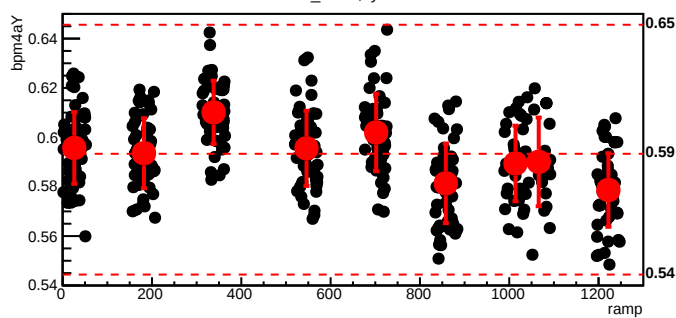
bmod_trim3,cyc=5167
