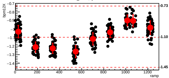
bmod_trim3,cyc=5167
