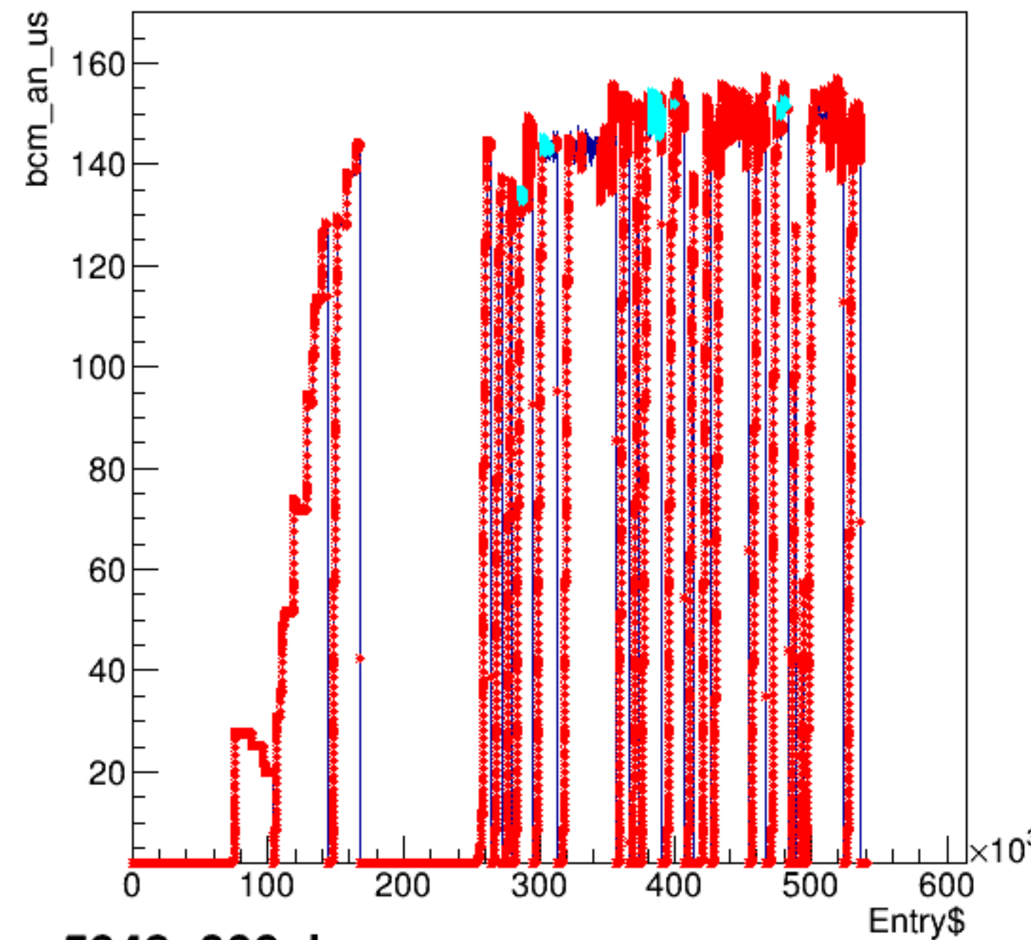
bcm_an_us:Entry$
