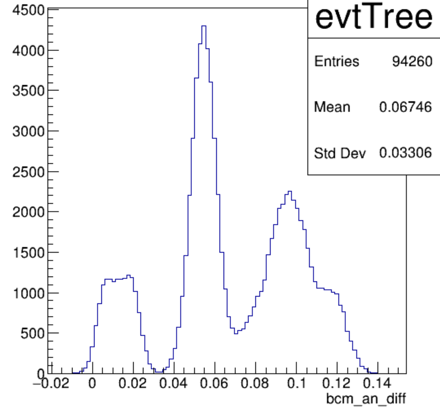
bcm_an_diff {ErrorFlag==0}
