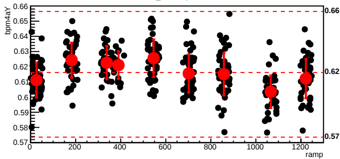
bmod_trim3,cyc=5248
