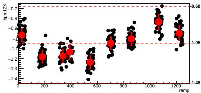
bmod_trim3,cyc=5248
