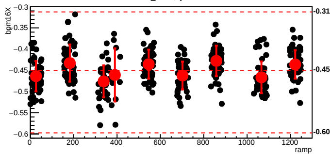
bmod_trim2,cyc=5252
