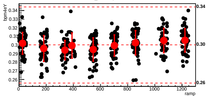
bmod_trim5,cyc=5252
