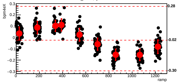
bmod_trim7,cyc=5252
