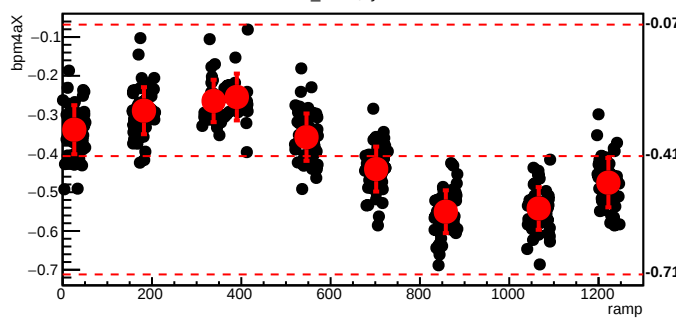
bmod_trim7,cyc=5252
