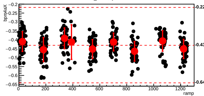
bmod_trim2,cyc=5252
