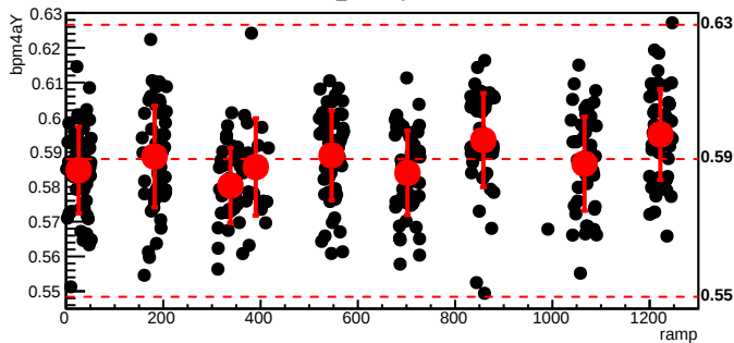
bmod_trim5,cyc=5252
