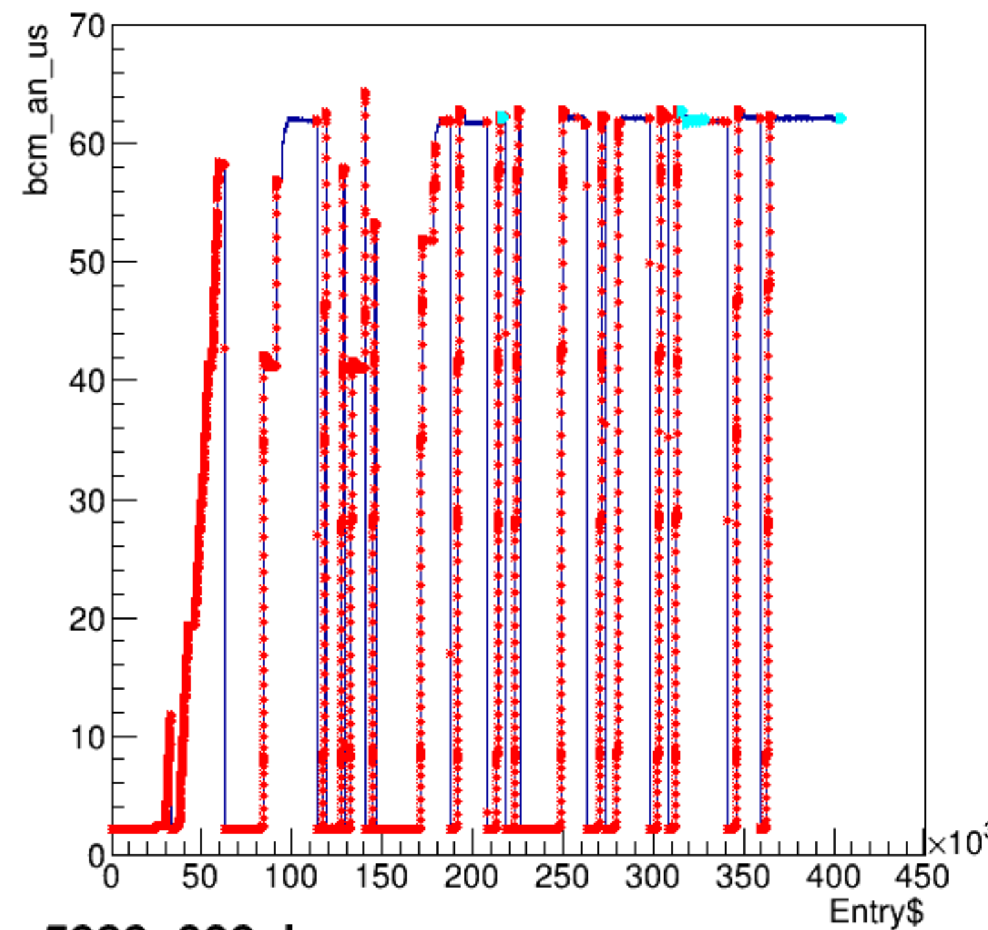
bcm_an_us:Entry$
