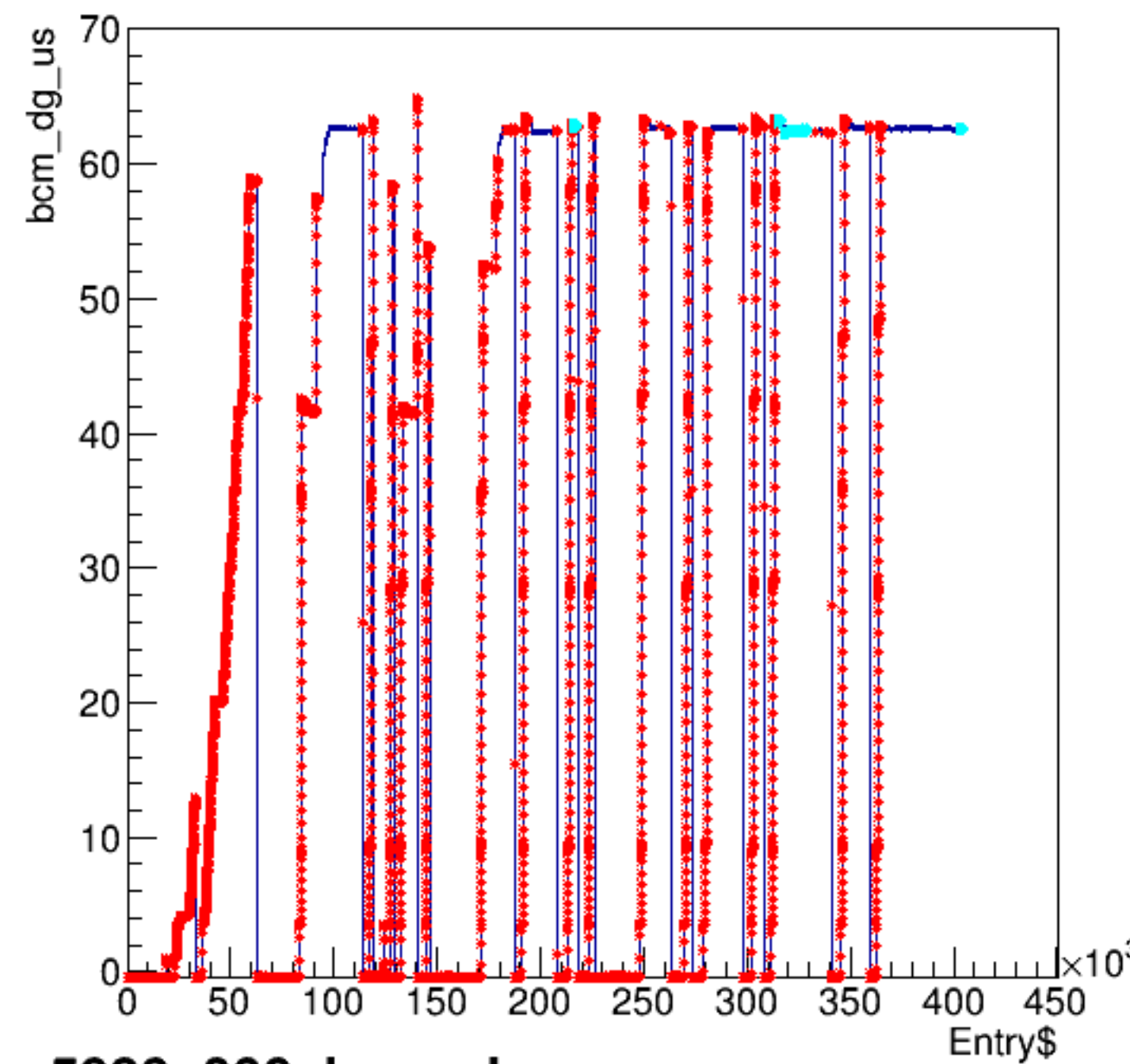
bcm_dg_us:Entry$
