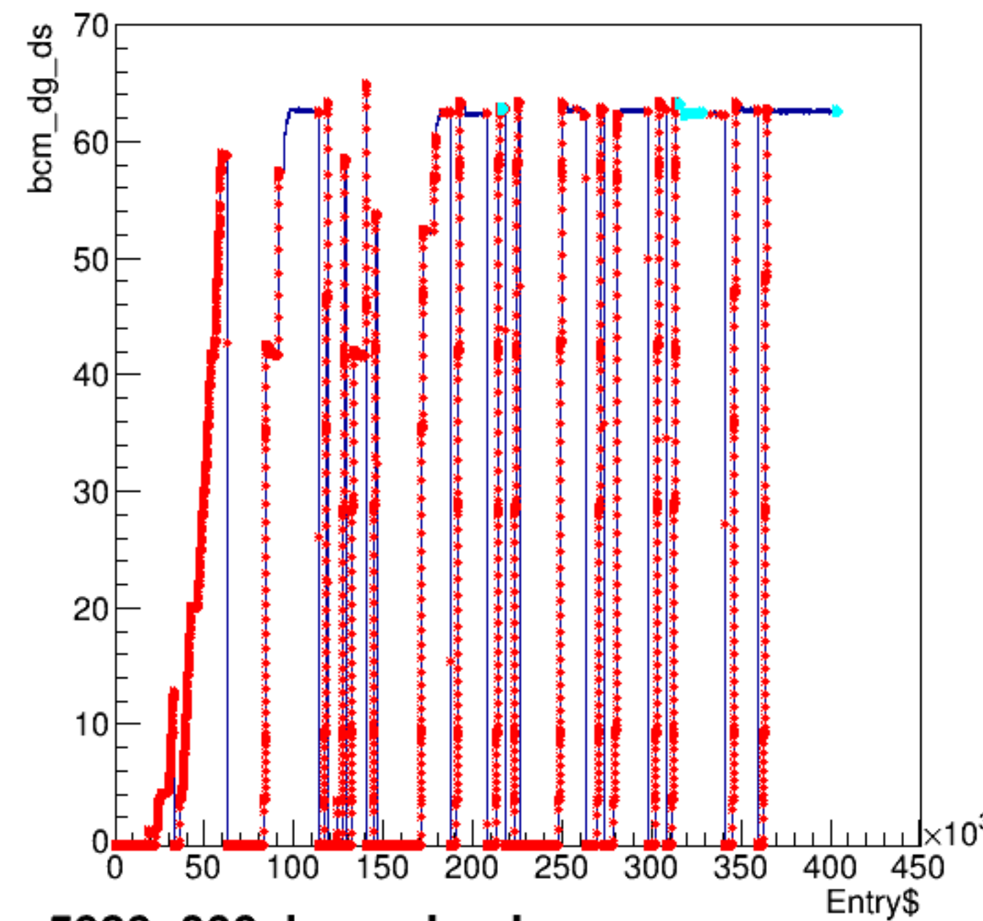
bcm_dg_ds:Entry$
