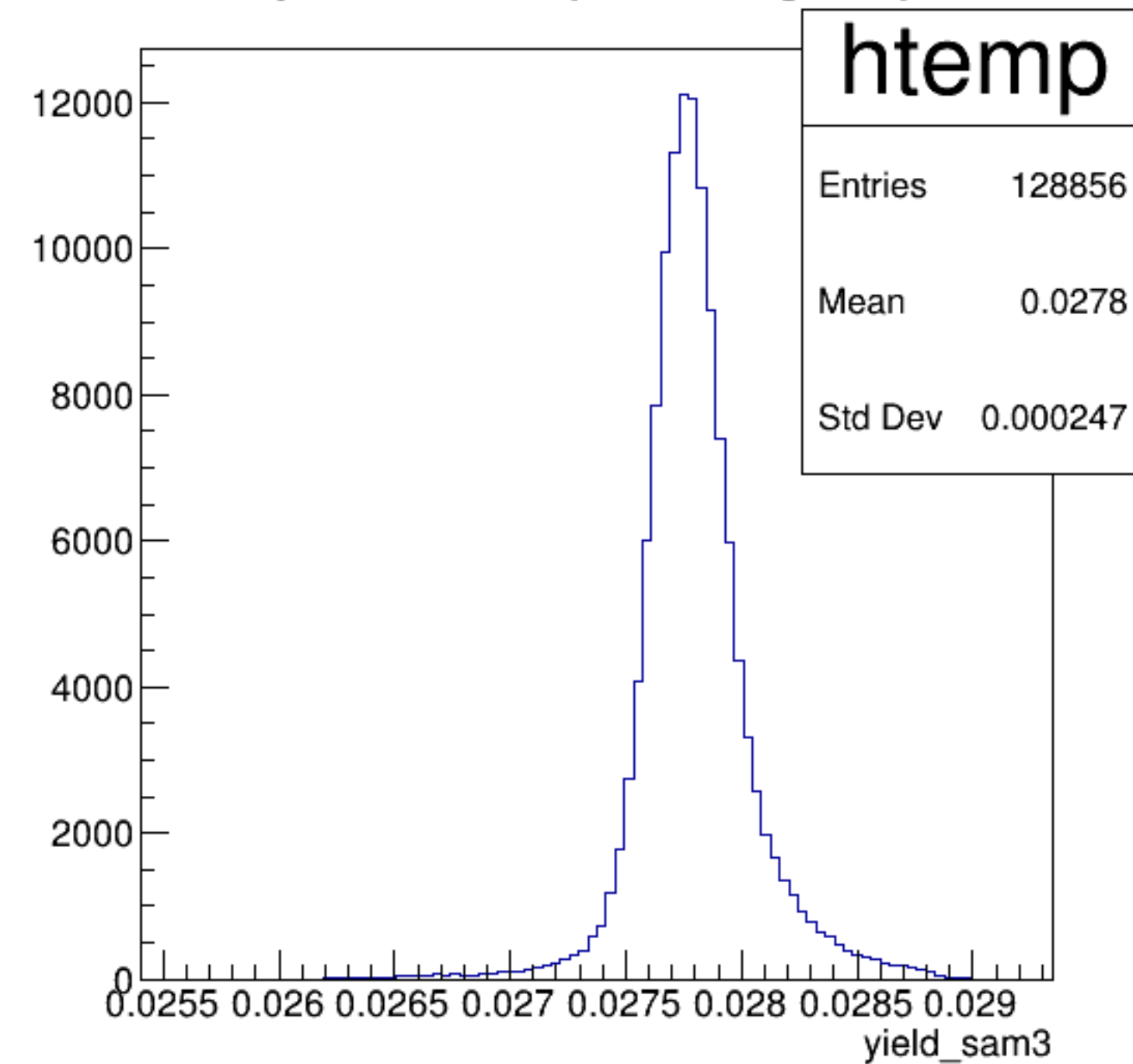
yield_sam3 {ErrorFlag==0}
