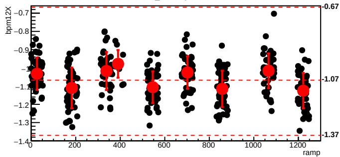
bmod_trim6,cyc=5200
