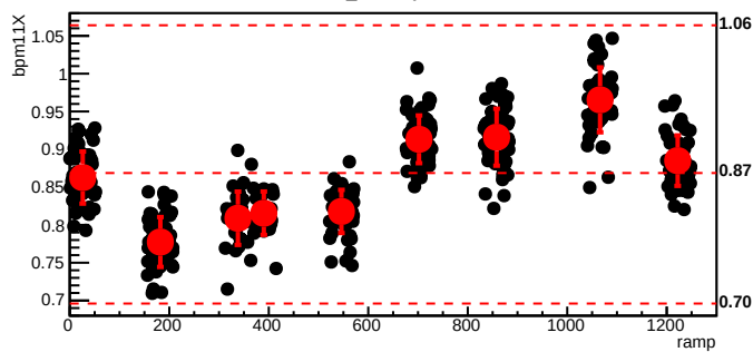
bmod_trim1,cyc=5200
