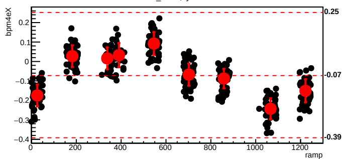
bmod_trim5,cyc=5200
