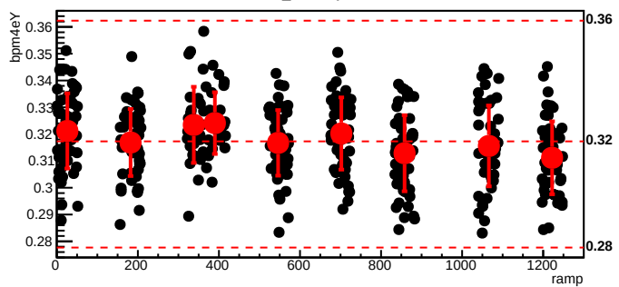
bmod_trim1,cyc=5200
