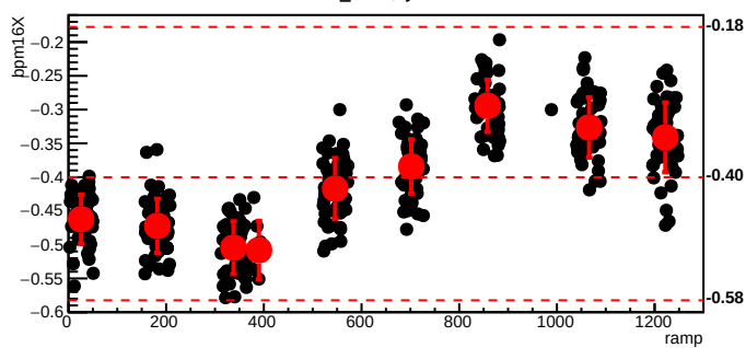
bmod_trim7,cyc=5200
