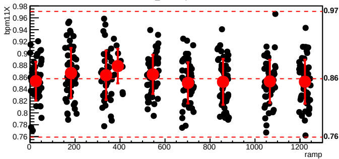
bmod_trim6,cyc=5200
