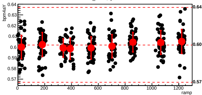
bmod_trim5,cyc=5200
