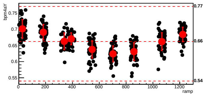
bmod_trim6,cyc=5265
