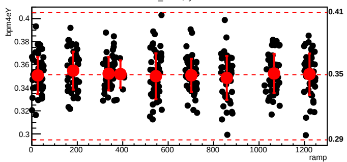
bmod_trim7,cyc=5265
