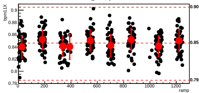
bmod_trim7,cyc=5265
