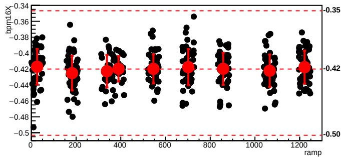
bmod_trim6,cyc=5265
