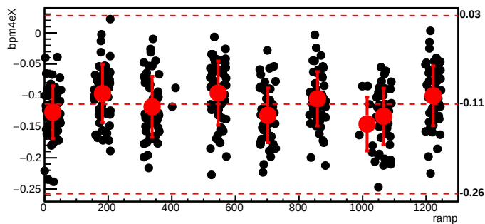
bmod_trim2,cyc=5270
