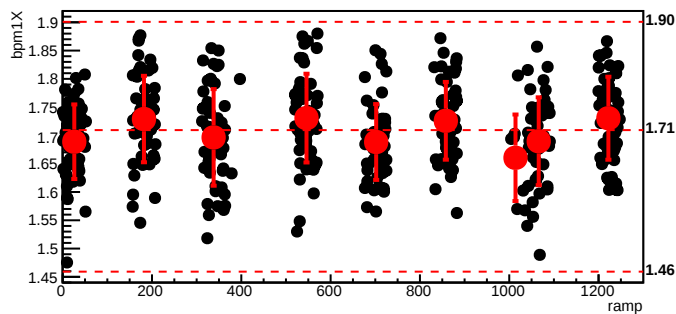
bmod_trim2,cyc=5270
