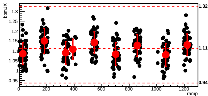
bmod_trim6,cyc=5270
