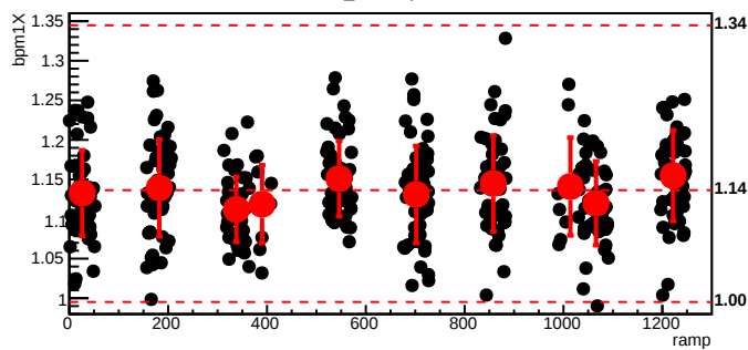
bmod_trim7,cyc=5270
