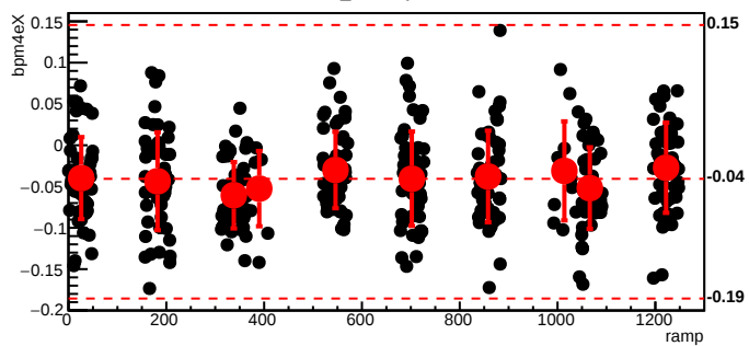
bmod_trim7,cyc=5270
