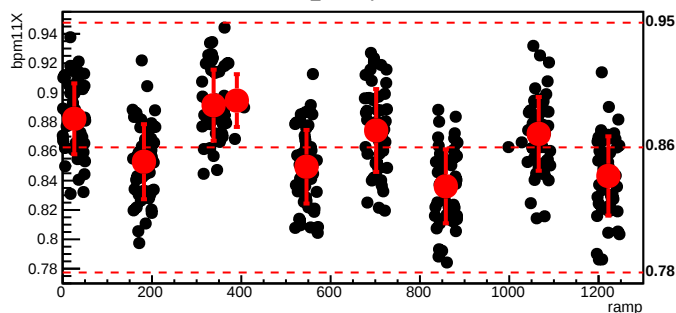
bmod_trim6,cyc=5270
