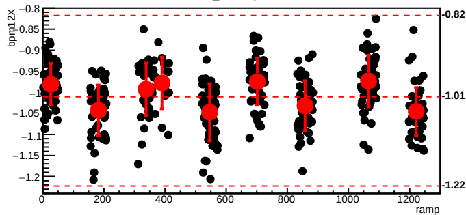
bmod_trim4,cyc=5270
