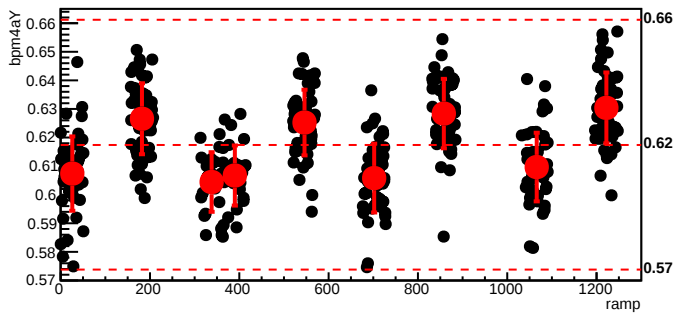
bmod_trim5,cyc=5270
