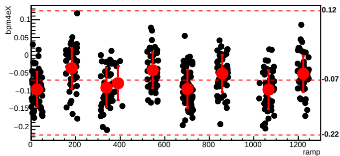
bmod_trim6,cyc=5270
