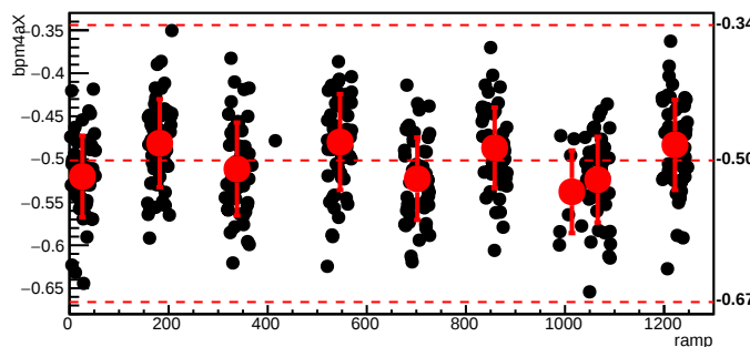
bmod_trim2,cyc=5270
