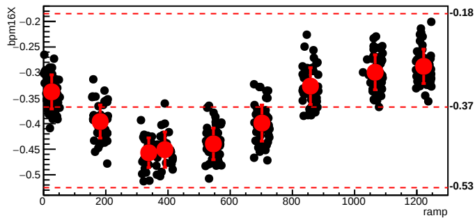
bmod_trim5,cyc=5270
