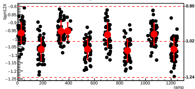
bmod_trim6,cyc=5270
