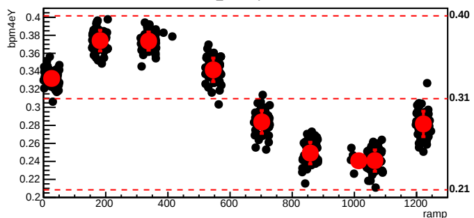
bmod_trim2,cyc=5270
