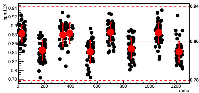
bmod_trim4,cyc=5270
