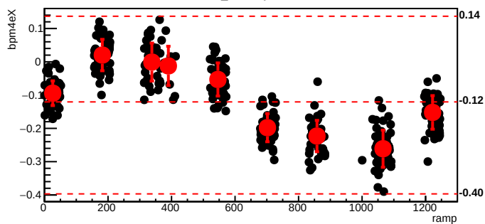
bmod_trim7,cyc=5278
