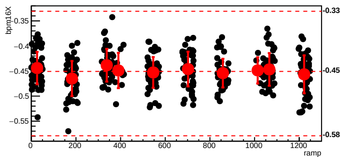
bmod_trim2,cyc=5278
