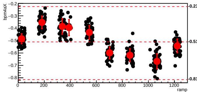
bmod_trim7,cyc=5278
