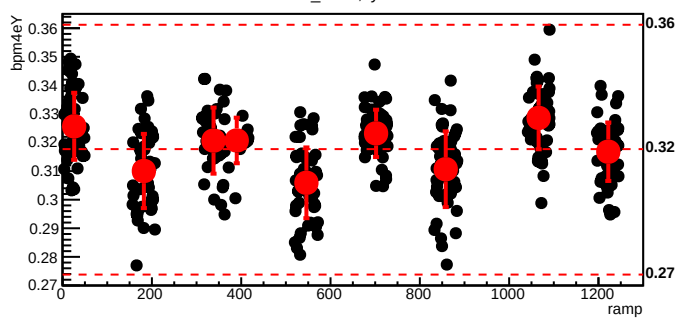
bmod_trim5,cyc=5278
