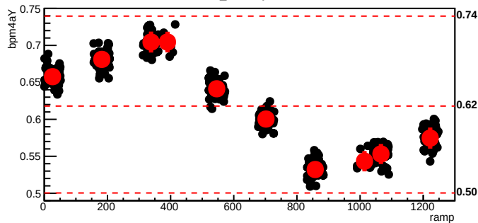
bmod_trim2,cyc=5278
