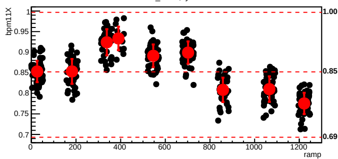
bmod_trim5,cyc=5278
