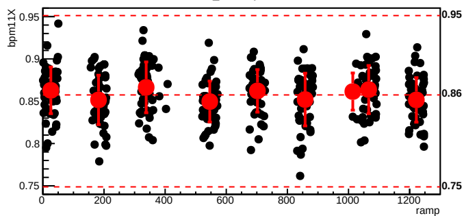
bmod_trim4,cyc=5278
