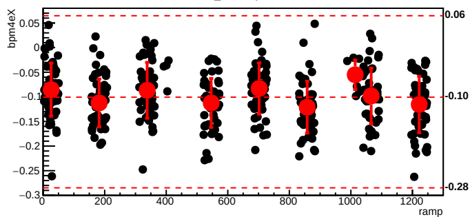
bmod_trim4,cyc=5278
