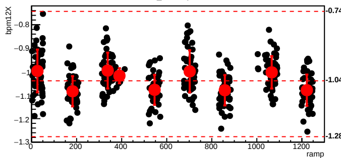
bmod_trim5,cyc=5290
