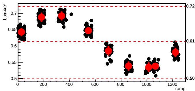
bmod_trim2,cyc=5290
