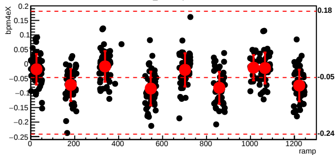
bmod_trim2,cyc=5290
