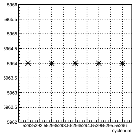
run:cyclenum {run == 5964}
