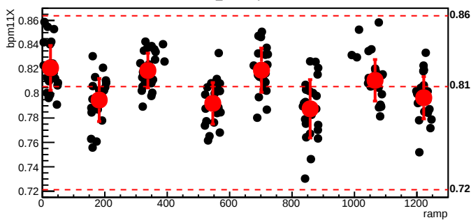
bmod_trim4,cyc=5295
