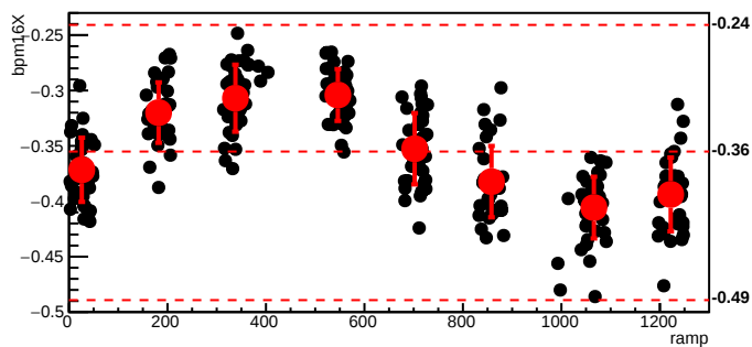
bmod_trim3,cyc=5295
