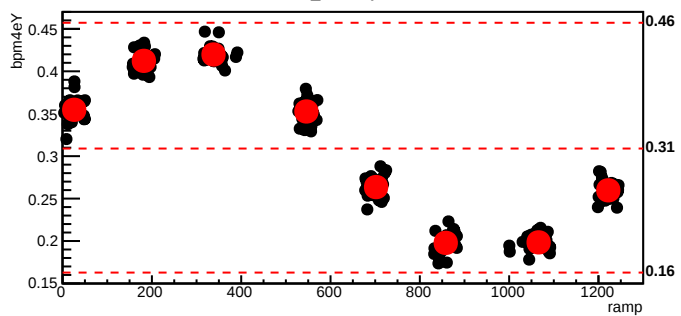
bmod_trim4,cyc=5295
