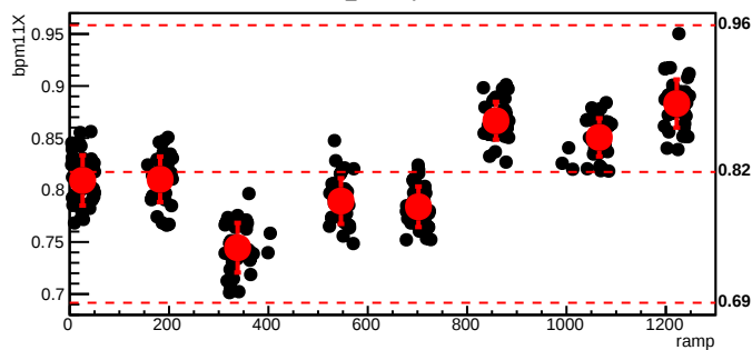
bmod_trim3,cyc=5295
