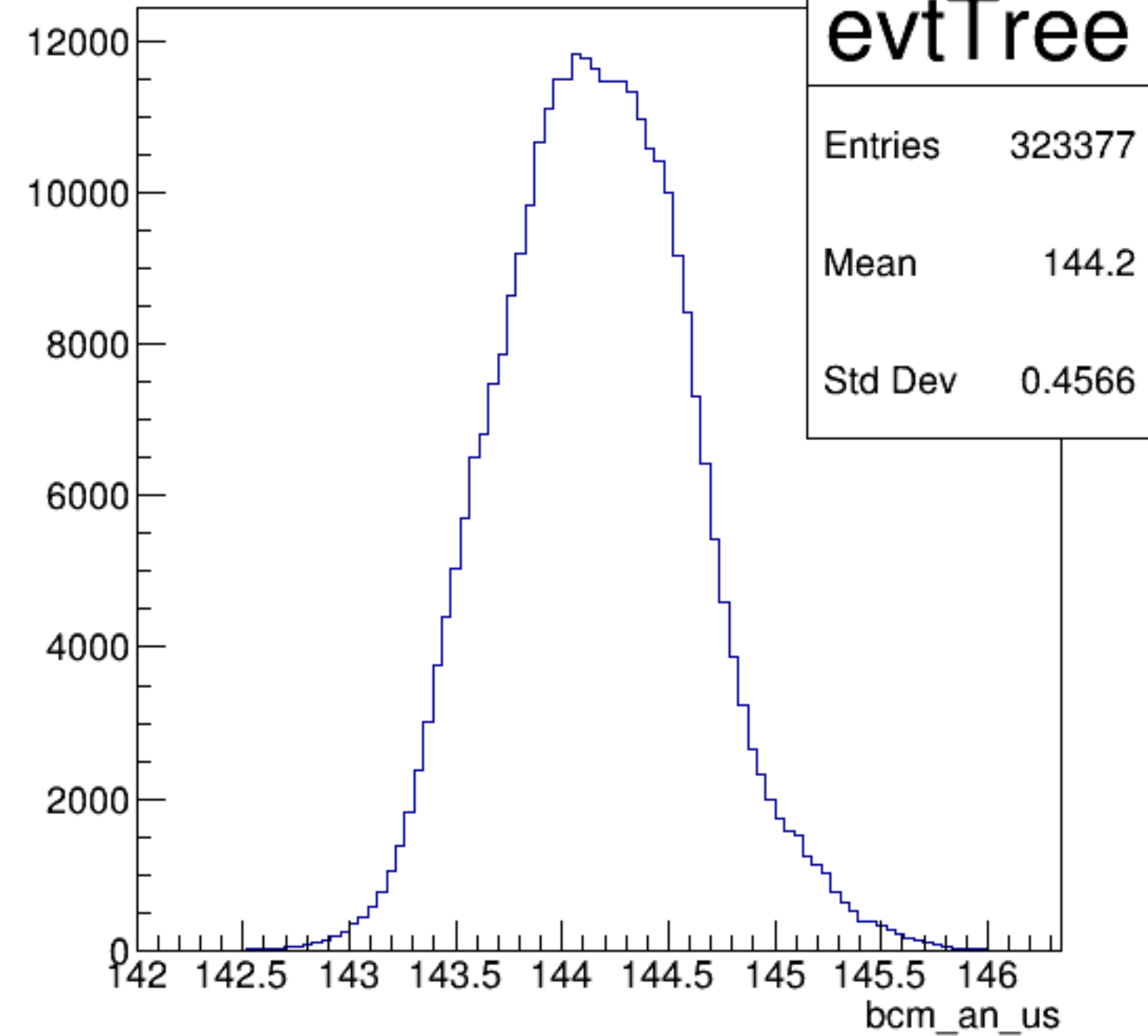
bcm_an_us {ErrorFlag==0}
