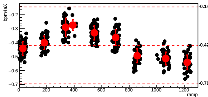
bmod_trim5,cyc=5303
