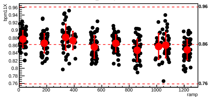
bmod_trim6,cyc=5303
