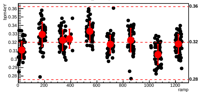
bmod_trim3,cyc=5303
