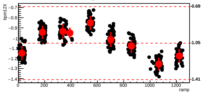
bmod_trim5,cyc=5303
