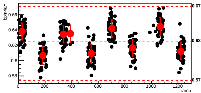
bmod_trim7,cyc=5303
