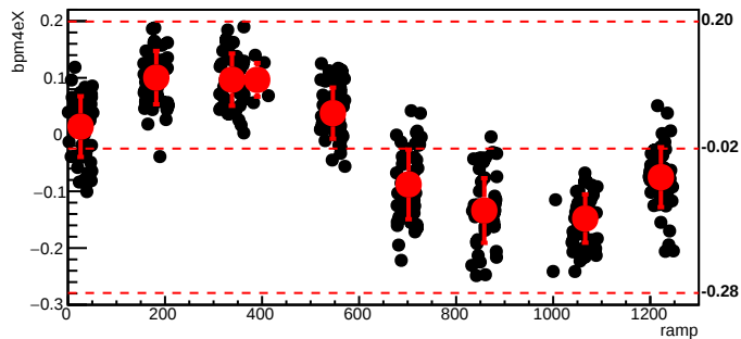
bmod_trim7,cyc=5303
