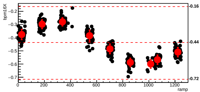
bmod_trim1,cyc=5303
