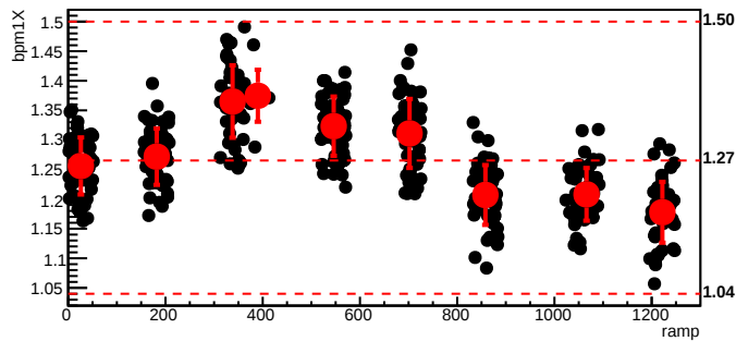
bmod_trim5,cyc=5303
