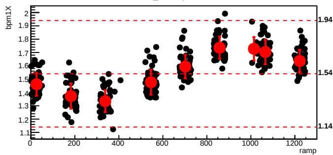
bmod_trim1,cyc=5303
