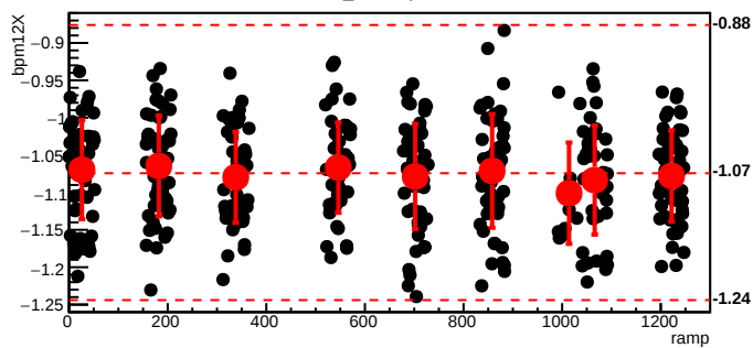
bmod_trim2,cyc=5303
