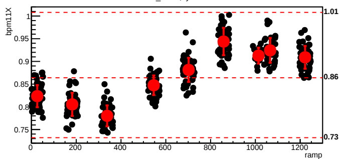
bmod_trim1,cyc=5305
