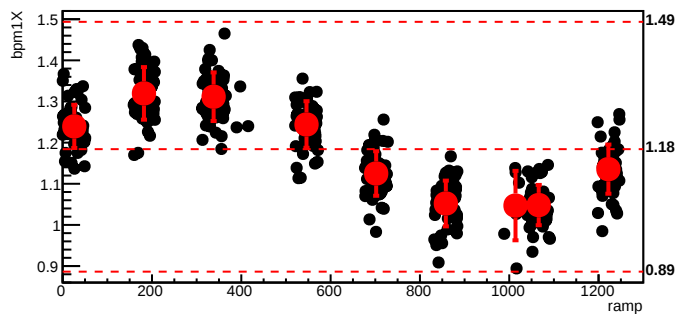
bmod_trim7,cyc=5305
