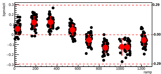
bmod_trim7,cyc=5305
