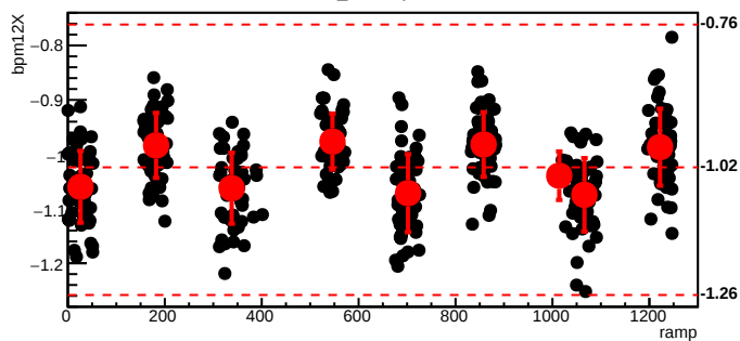
bmod_trim2,cyc=5305
