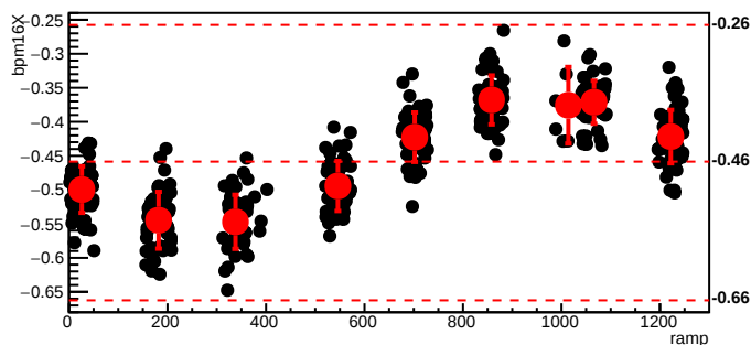
bmod_trim7,cyc=5305
