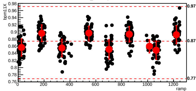
bmod_trim2,cyc=5305
