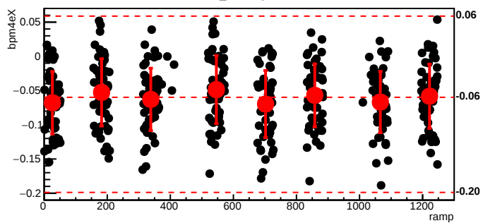
bmod_trim4,cyc=5305
