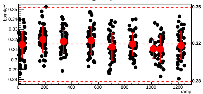
bmod_trim1,cyc=5305
