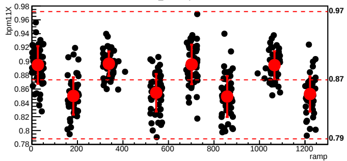
bmod_trim4,cyc=5305
