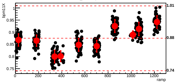
bmod_trim3,cyc=5305
