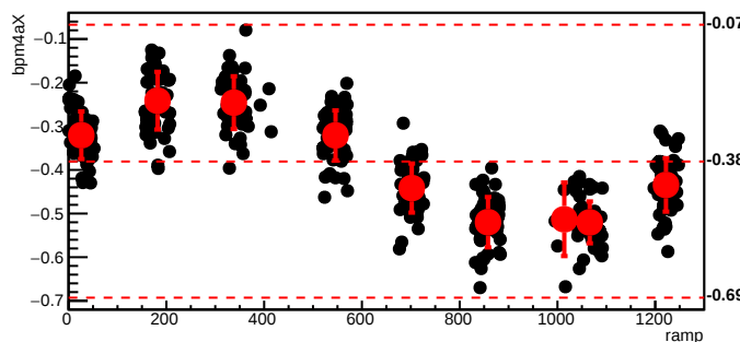
bmod_trim7,cyc=5305
