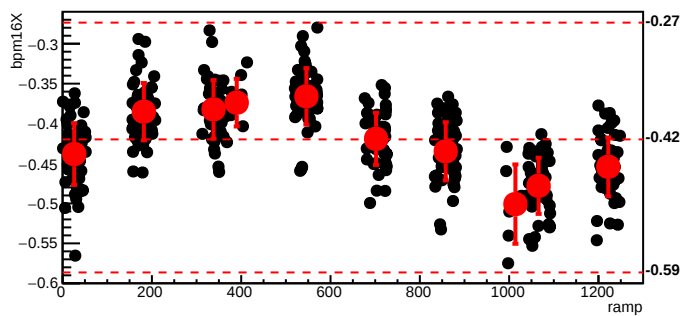
bmod_trim3,cyc=5305
