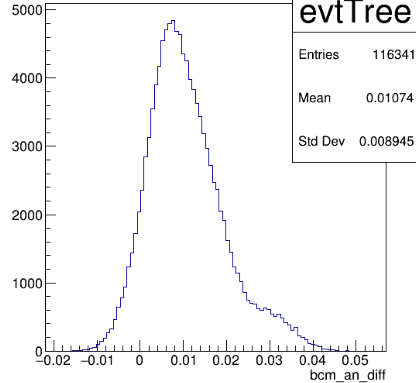
bcm_an_diff {ErrorFlag==0}
