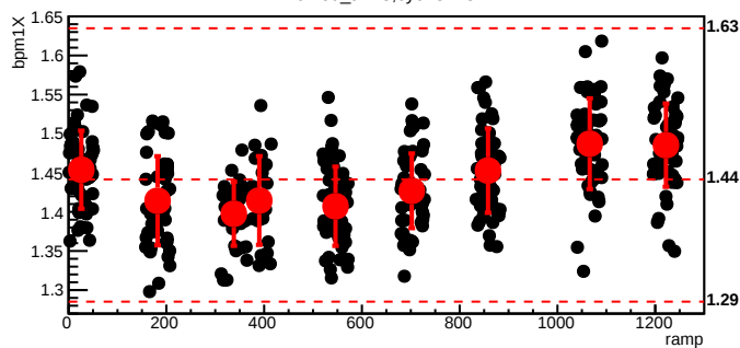
bmod_trim3,cyc=5418
