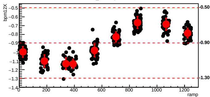
bmod_trim7,cyc=5418
