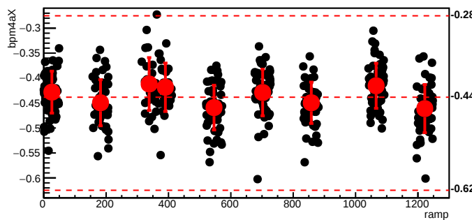
bmod_trim4,cyc=5418
