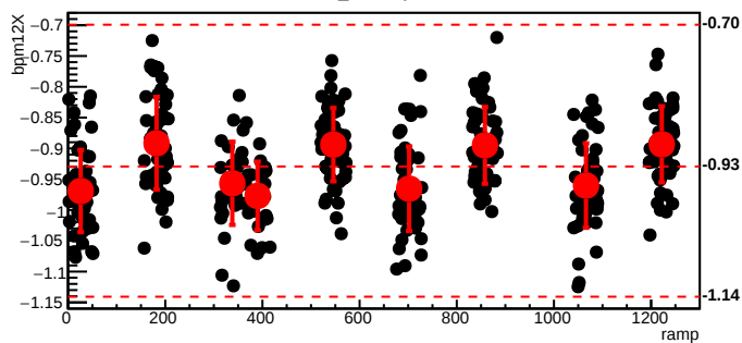
bmod_trim4,cyc=5418
