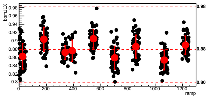
bmod_trim6,cyc=5420
