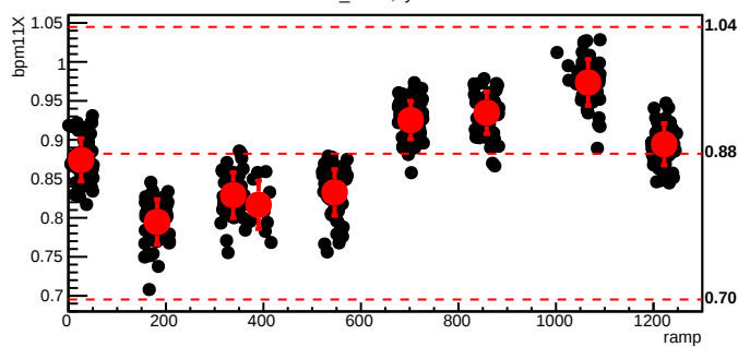
bmod_trim1,cyc=5420
