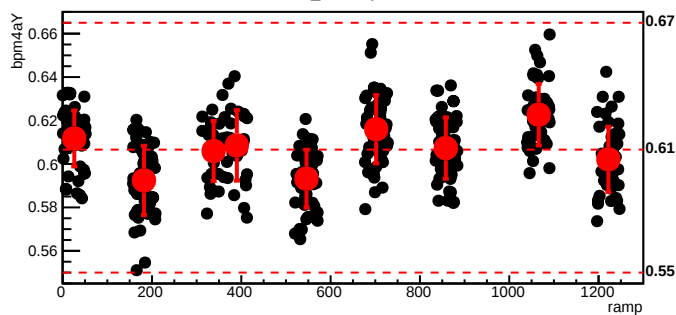
bmod_trim7,cyc=5420
