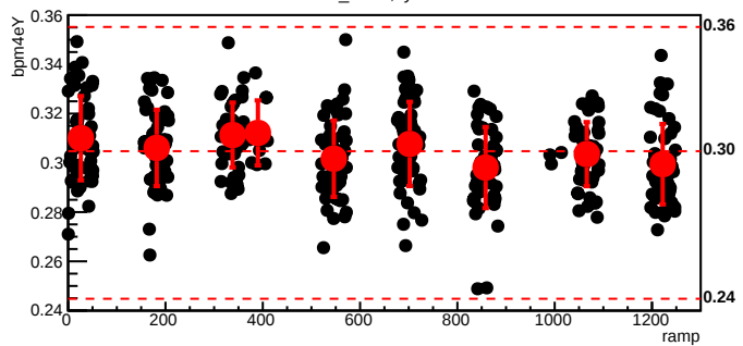
bmod_trim1,cyc=5420
