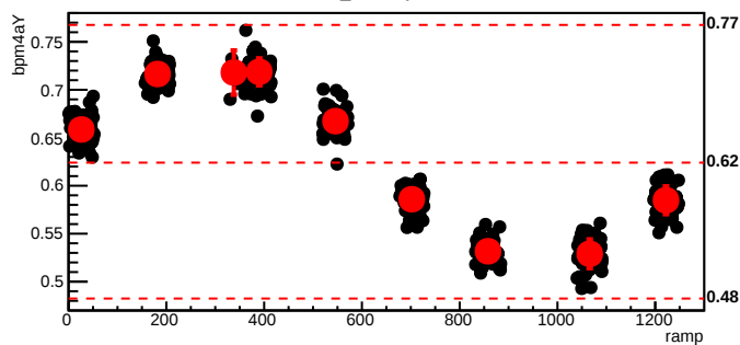
bmod_trim2,cyc=5422
