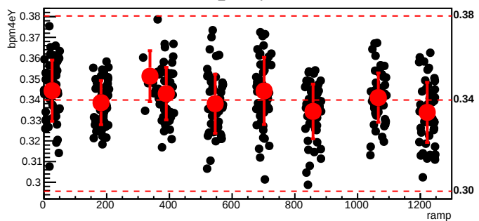
bmod_trim1,cyc=5422
