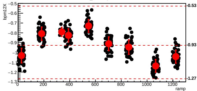
bmod_trim5,cyc=5422
