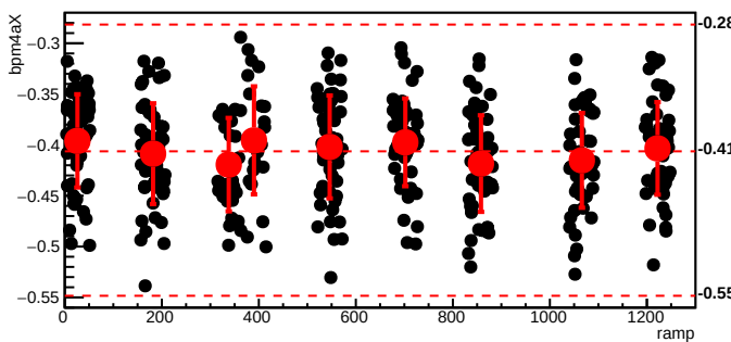
bmod_trim2,cyc=5479
