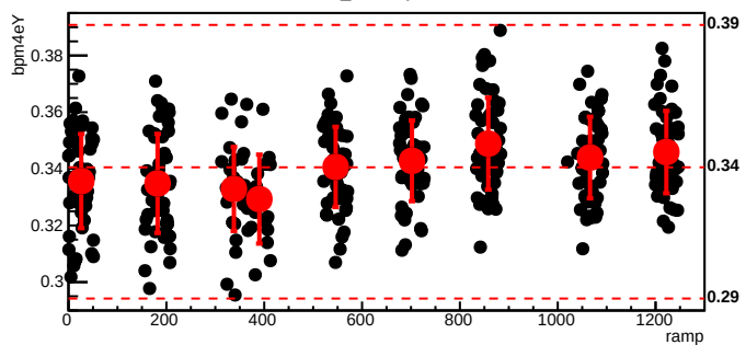
bmod_trim7,cyc=5479
