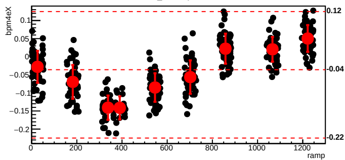
bmod_trim3,cyc=5479
