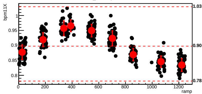
bmod_trim5,cyc=5479
