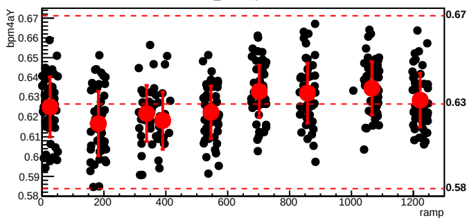
bmod_trim7,cyc=5479
