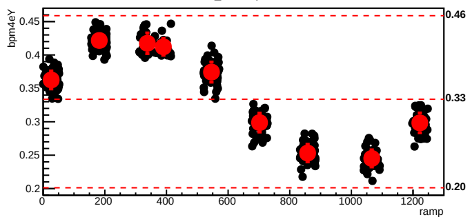
bmod_trim2,cyc=5479
