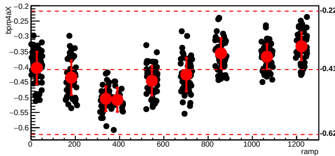
bmod_trim3,cyc=5479
