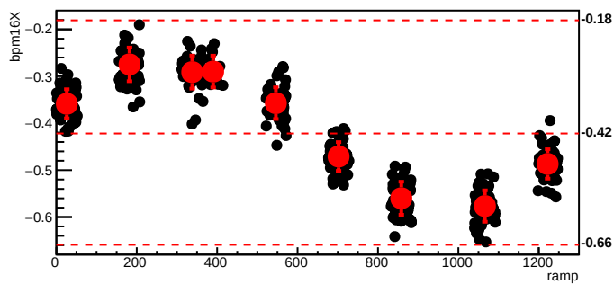
bmod_trim1,cyc=5479
