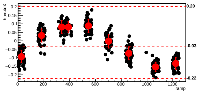
bmod_trim5,cyc=5479
