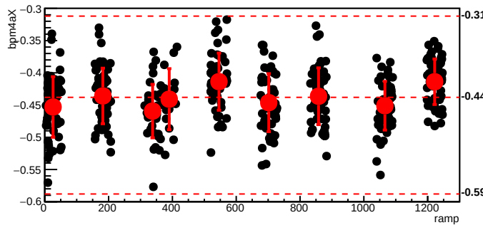
bmod_trim4,cyc=5479
