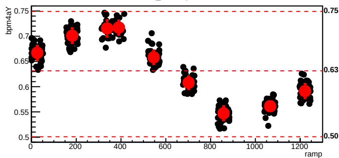
bmod_trim6,cyc=5479
