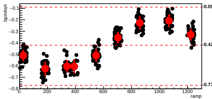
bmod_trim1,cyc=5479
