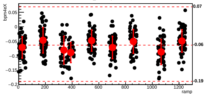
bmod_trim6,cyc=5479
