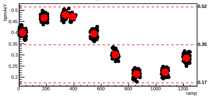
bmod_trim4,cyc=5479
