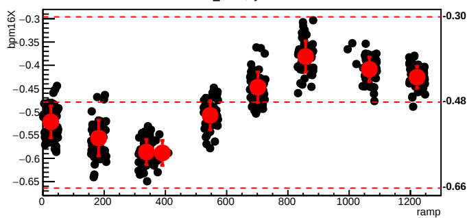
bmod_trim7,cyc=5476
