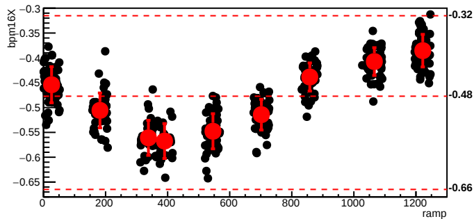
bmod_trim5,cyc=5476
