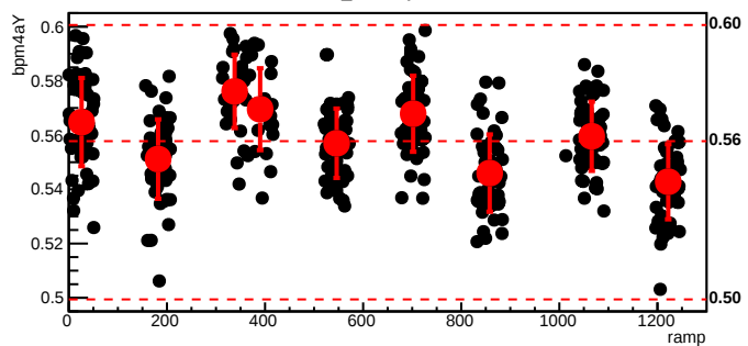
bmod_trim3,cyc=5476
