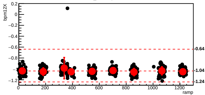
bmod_trim4,cyc=5476
