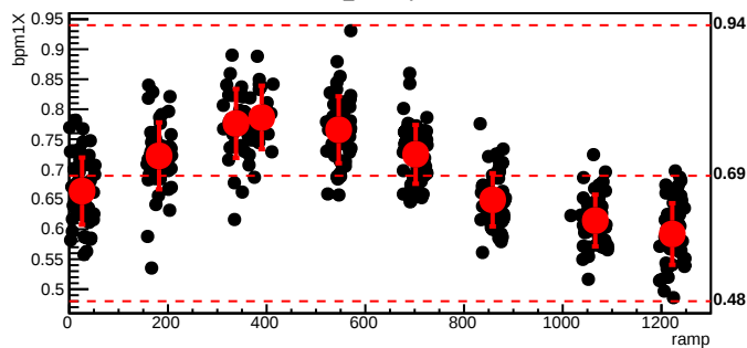
bmod_trim5,cyc=5476
