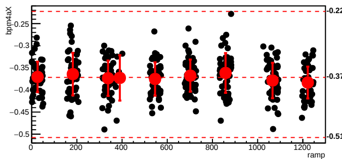
bmod_trim2,cyc=5476
