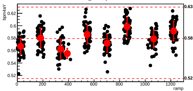
bmod_trim7,cyc=5476
