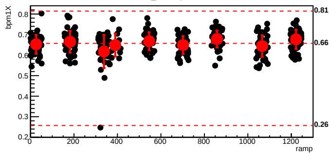
bmod_trim4,cyc=5476
