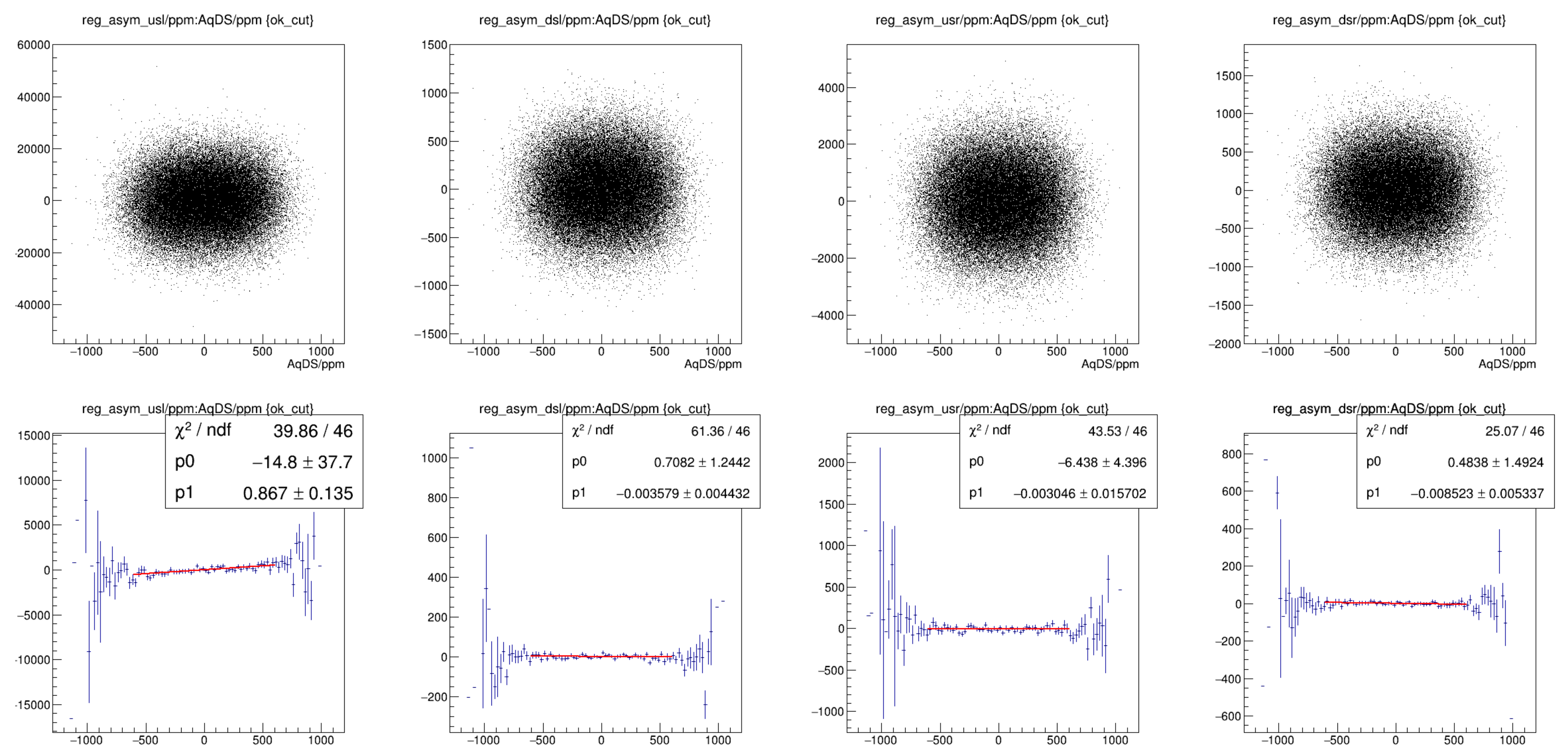
run6109_000_main_vs_AqDS_ratecheck_reg_postpan.png
