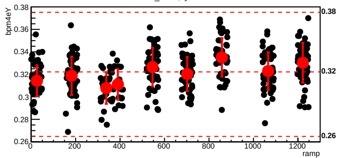
bmod_trim7,cyc=5518
