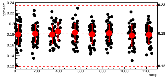
bmod_trim1,cyc=5515
