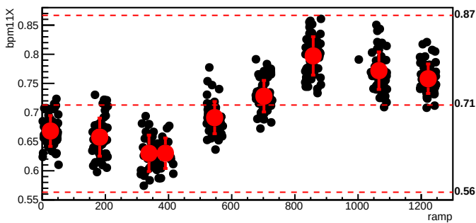
bmod_trim1,cyc=5515
