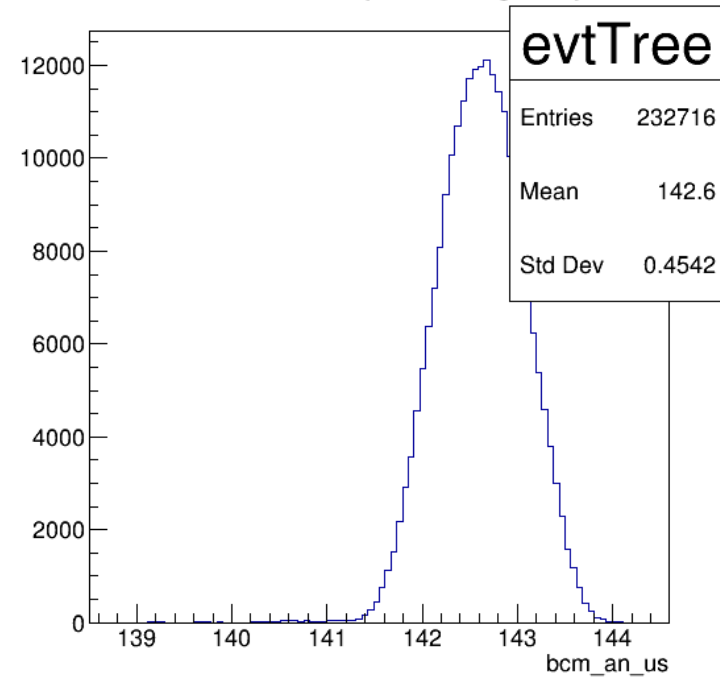
bcm_an_us {ErrorFlag==0}
