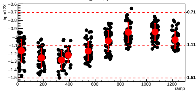
bmod_trim1,cyc=5643
