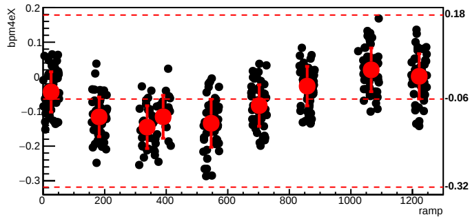
bmod_trim3,cyc=5643
