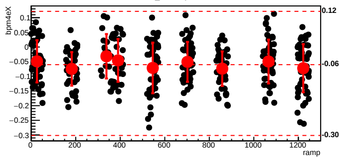
bmod_trim4,cyc=5643
