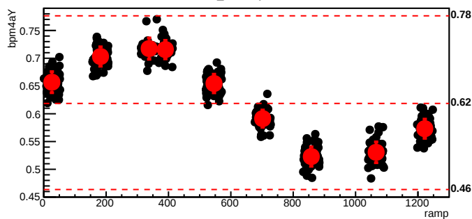
bmod_trim2,cyc=5643
