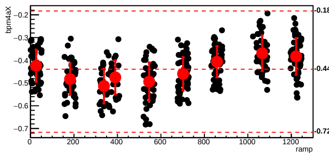
bmod_trim3,cyc=5643
