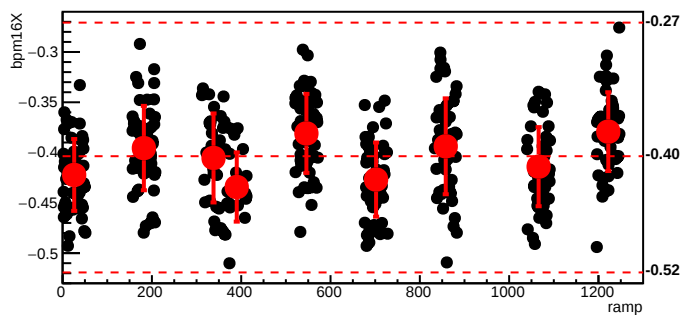
bmod_trim6,cyc=5643
