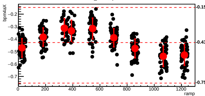
bmod_trim5,cyc=5643
