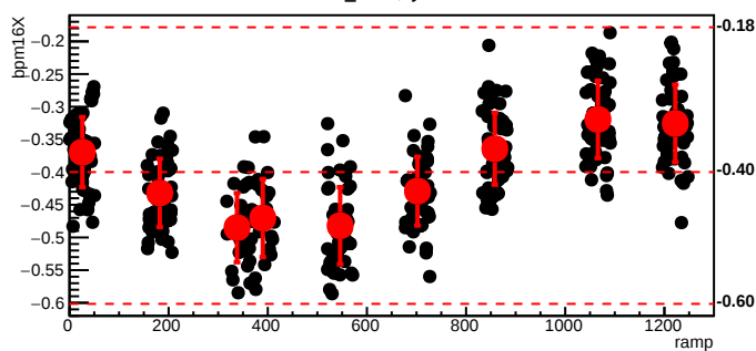
bmod_trim5,cyc=5643
