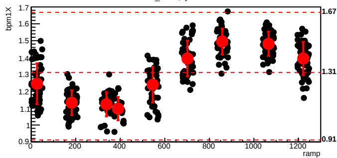
bmod_trim1,cyc=5643
