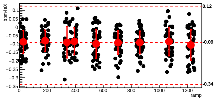
bmod_trim2,cyc=5643
