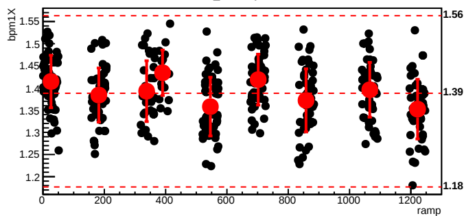
bmod_trim6,cyc=5643
