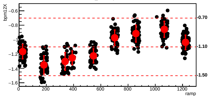
bmod_trim7,cyc=5643
