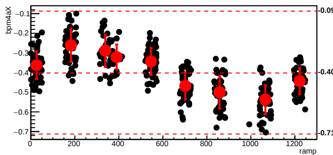
bmod_trim7,cyc=5643
