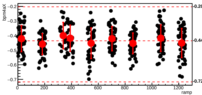
bmod_trim4,cyc=5643
