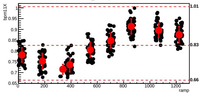
bmod_trim7,cyc=5653
