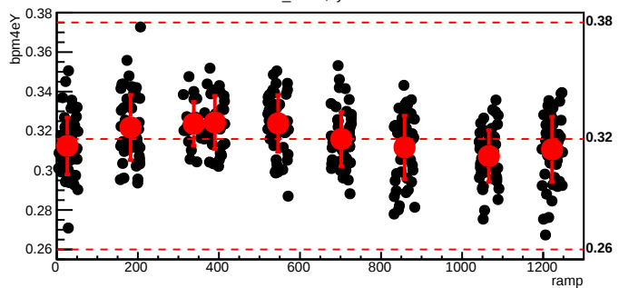
bmod_trim3,cyc=5653
