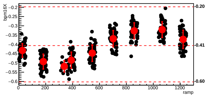
bmod_trim7,cyc=5653
