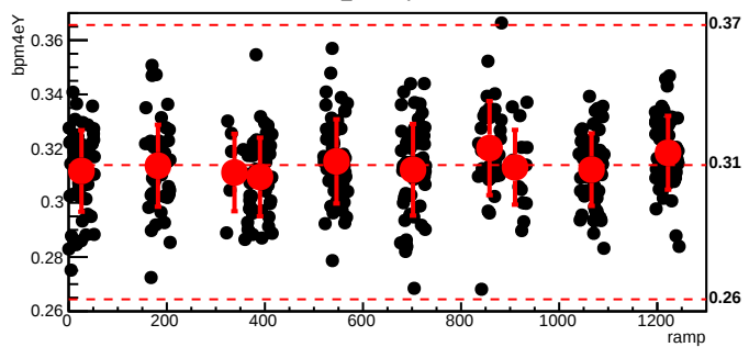
bmod_trim5,cyc=5653
