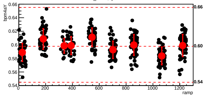
bmod_trim3,cyc=5653
