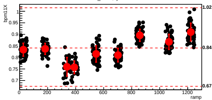
bmod_trim3,cyc=5653
