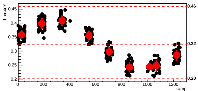
bmod_trim2,cyc=5692
