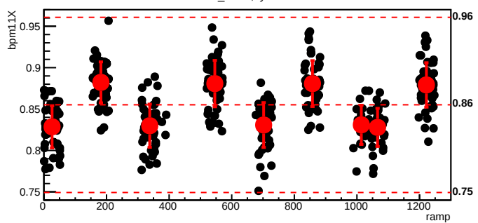
bmod_trim4,cyc=5692
