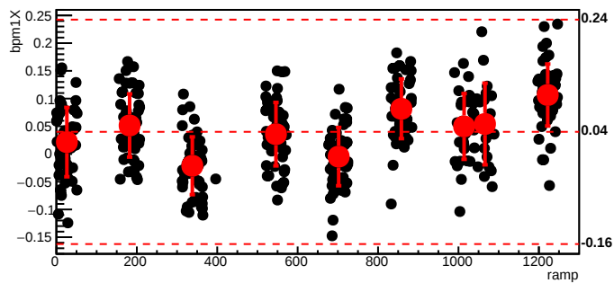
bmod_trim3,cyc=5692
