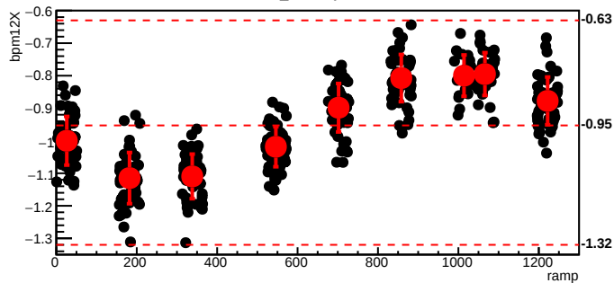
bmod_trim1,cyc=5692
