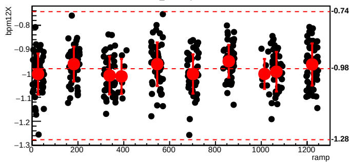
bmod_trim4,cyc=5695
