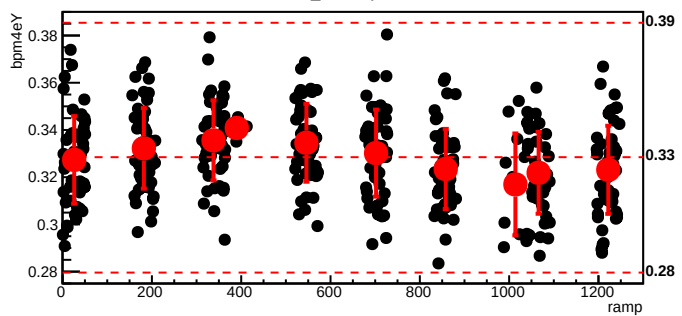
bmod_trim3,cyc=5695
