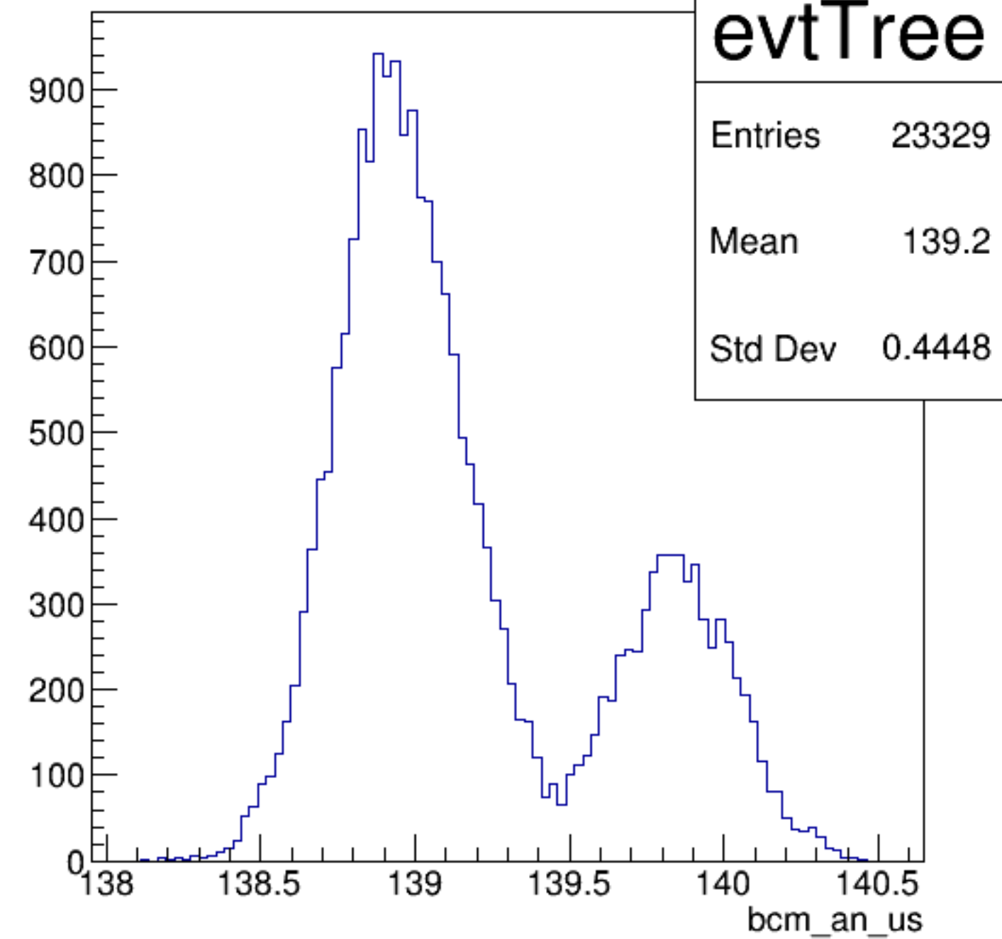
bcm_an_us {ErrorFlag==0}
