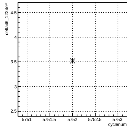
delta46_12X4eY:cyclenum {run == 6208}
