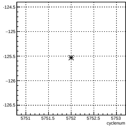
usr_4eY:cyclenum {run == 6208}
