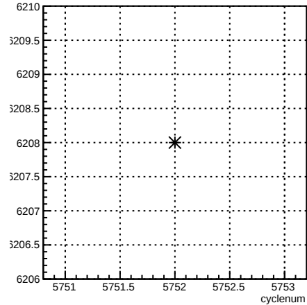
run:cyclenum {run == 6208}
