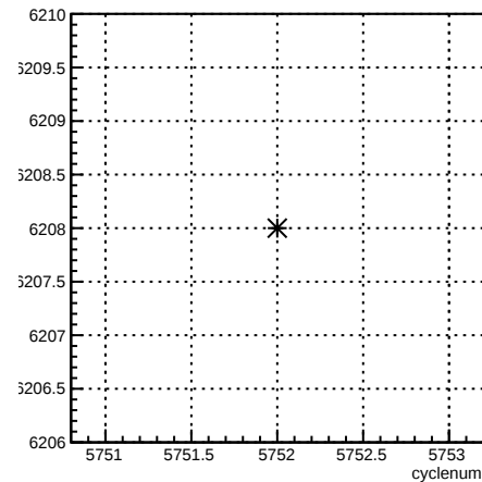
run:cyclenum {run == 6208}
