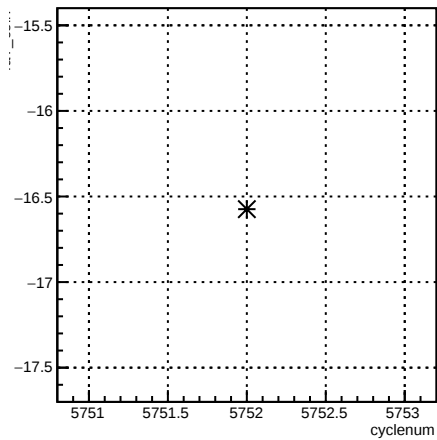
4eY_coil7:cyclenum {run == 6208}
