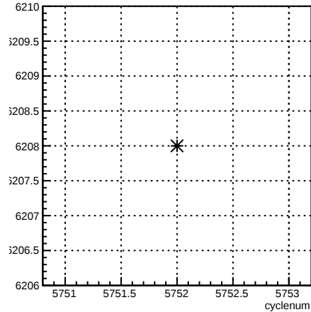
run:cyclenum {run == 6208}
