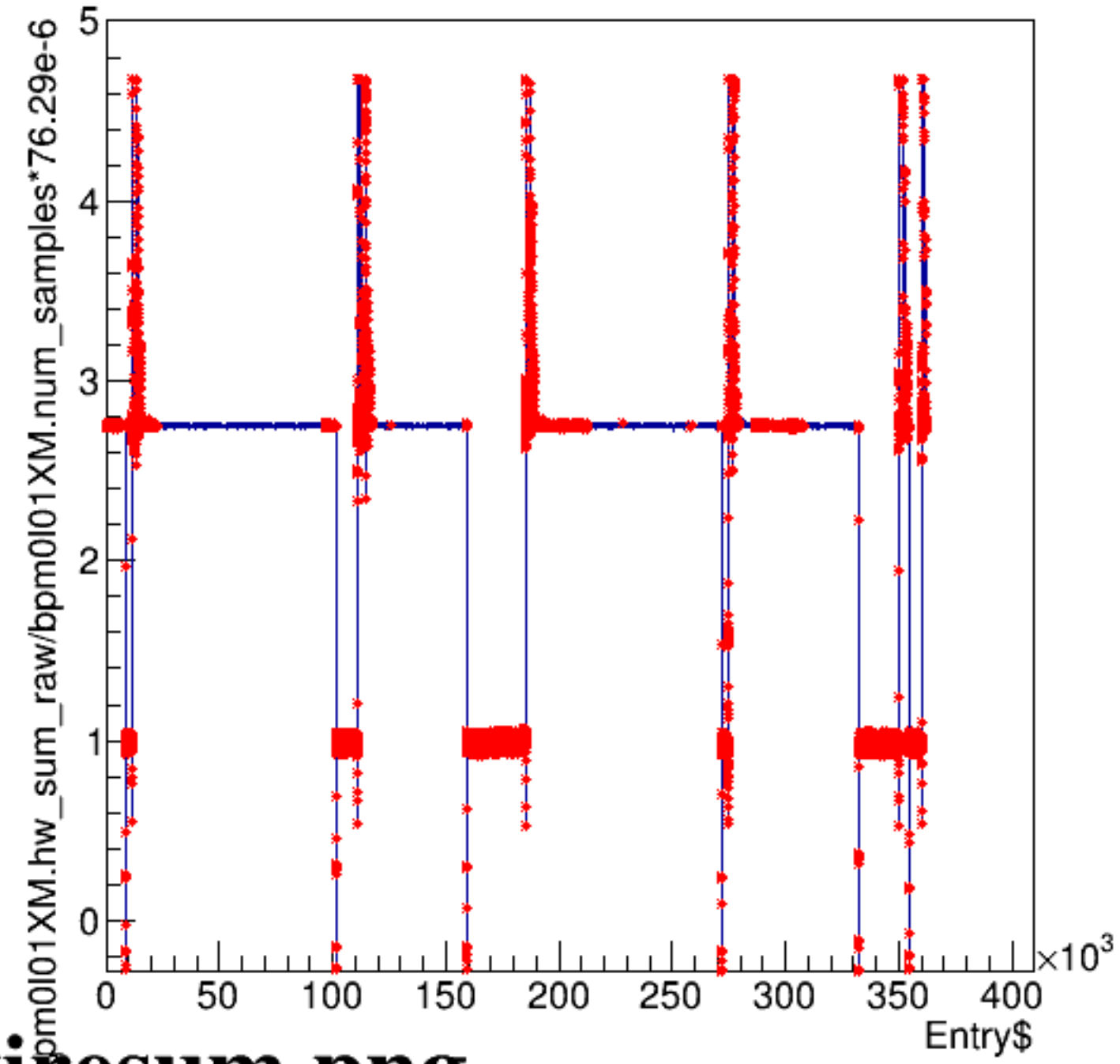
bpm0l01XM.hw_sum_raw/bpm0l01XM.num_samples*76.29e-6:Entry$
