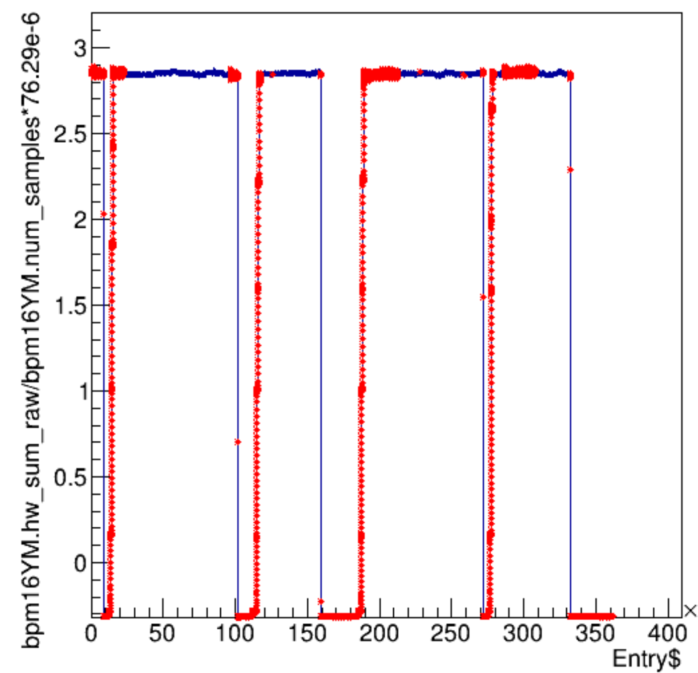
bpm16YM.hw_sum_raw/bpm16YM.num_samples*76.29e-6:Entry$
