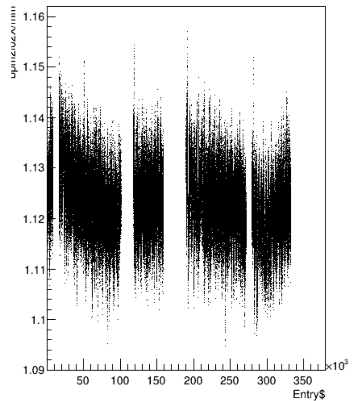
bpm2i02X/mm:Entry$ {ErrorFlag==0}
