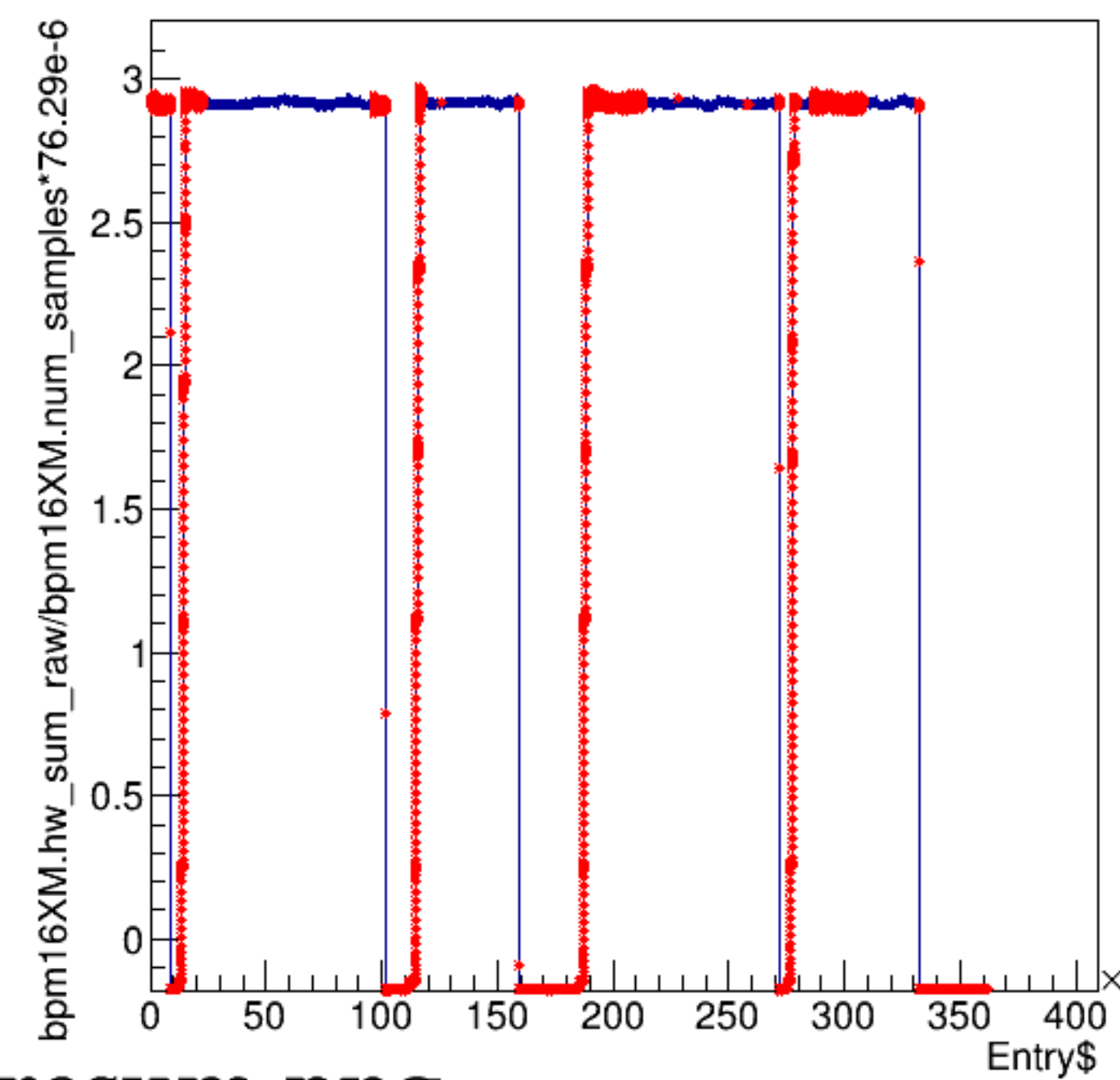
bpm16XM.hw_sum_raw/bpm16XM.num_samples*76.29e-6:Entry$
