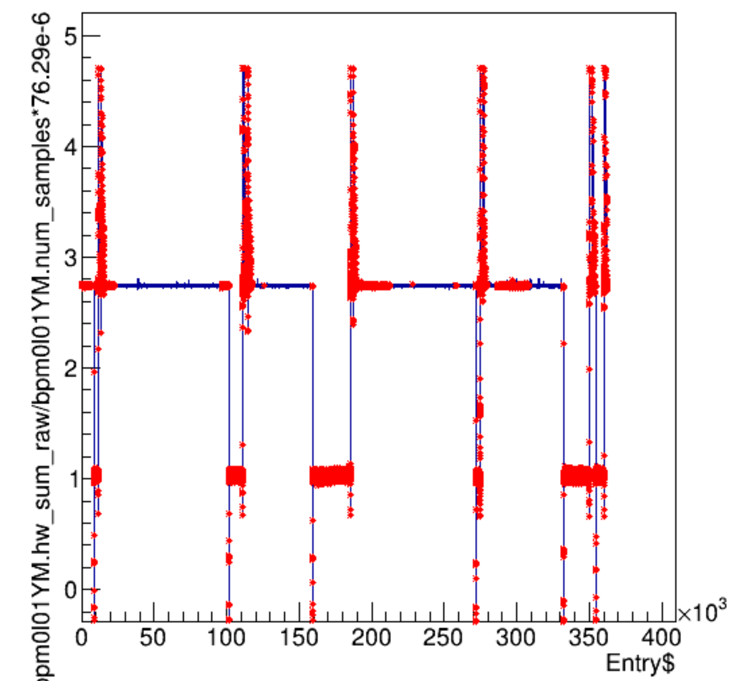
bpm0l01YM.hw_sum_raw/bpm0l01YM.num_samples*76.29e-6:Entry$
