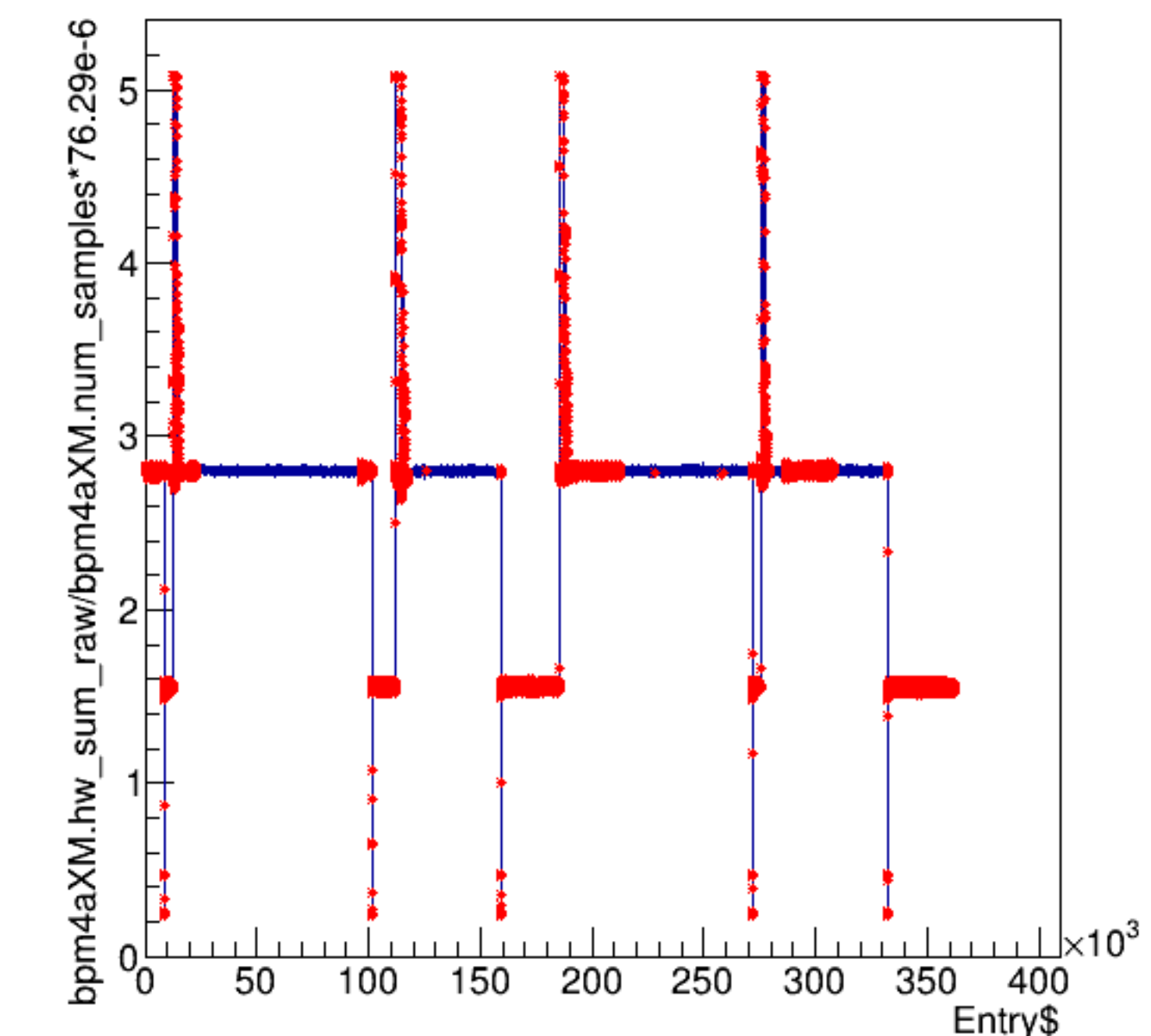
bpm4aXM.hw_sum_raw/bpm4aXM.num_samples*76.29e-6:Entry$
