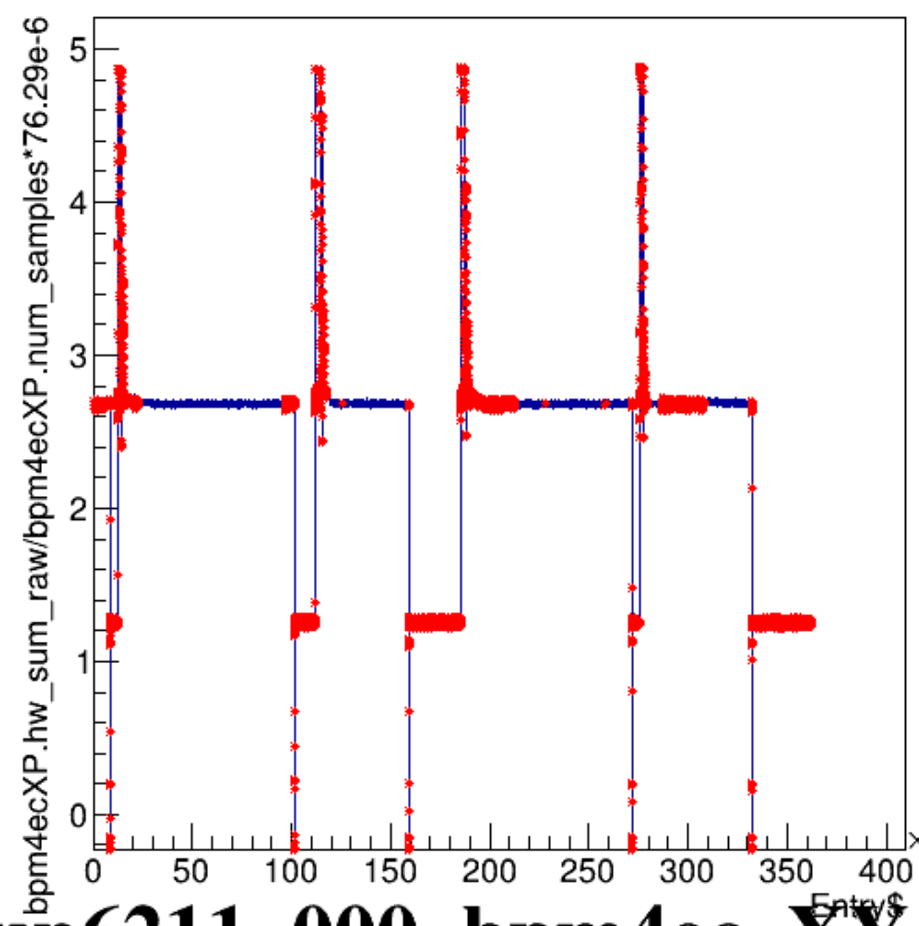
bpm4ecXP.hw_sum_raw/bpm4ecXP.num_samples*76.29e-6:Entry$
