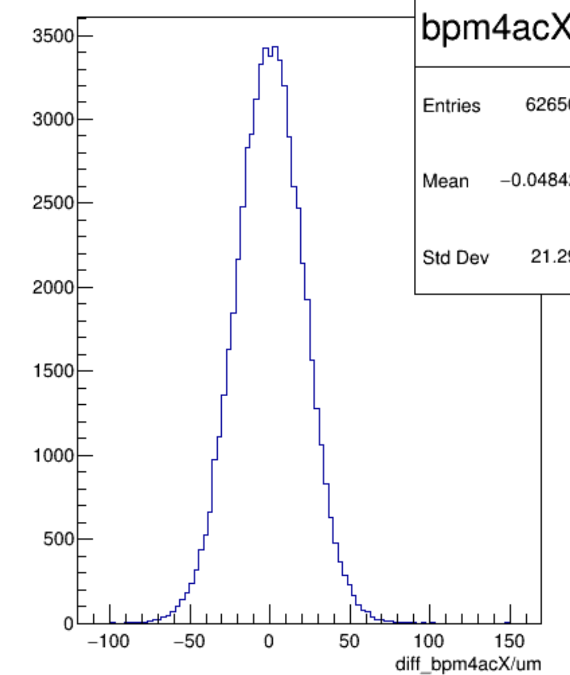
diff_bpm4acX/um {ErrorFlag==0}
