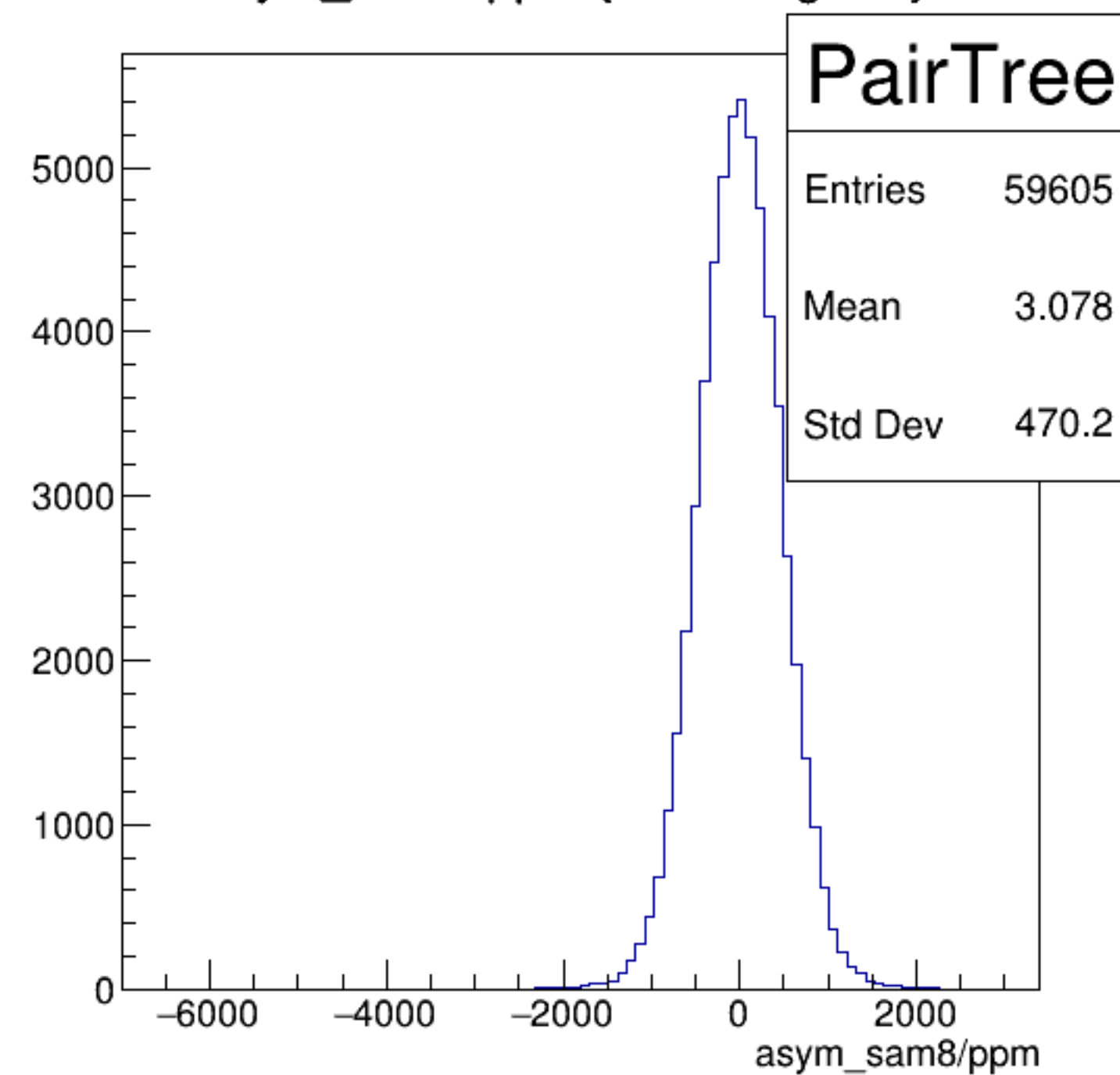
asym_sam8/ppm {ErrorFlag==0}
