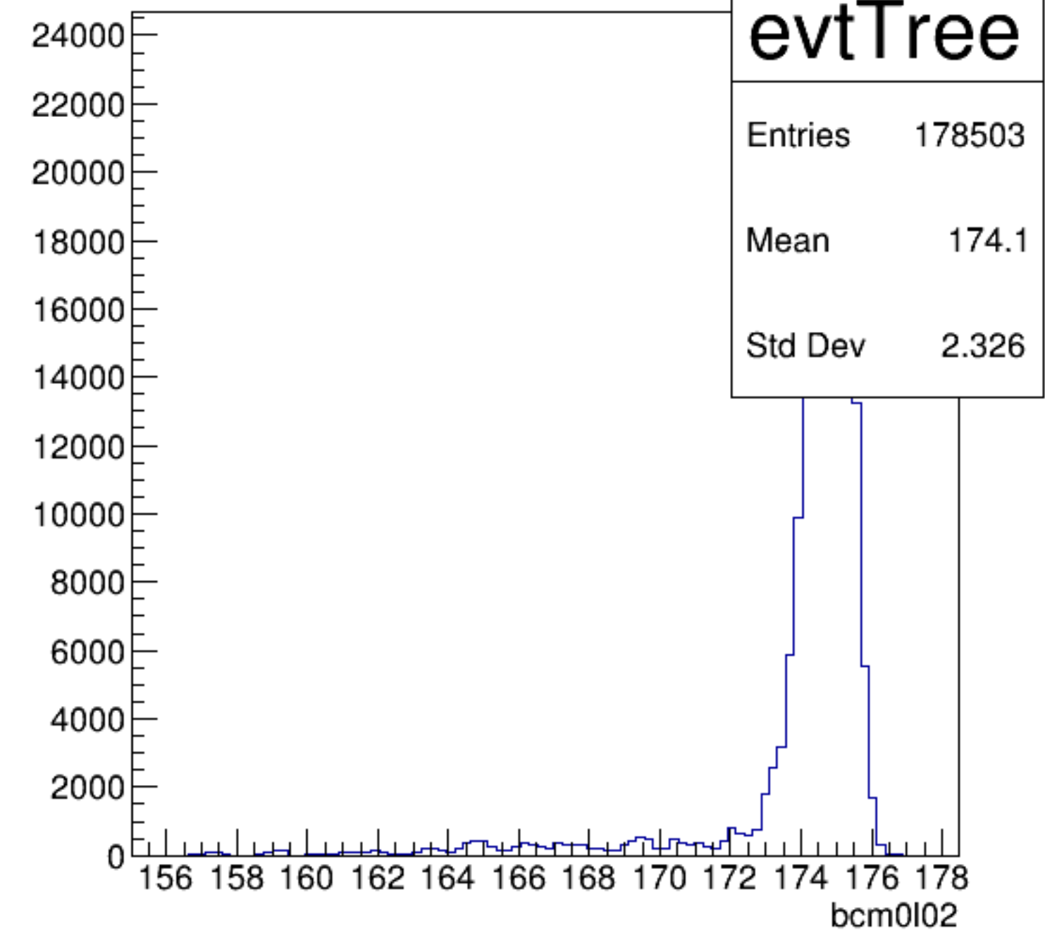
bcm0l02 {ErrorFlag==0}
