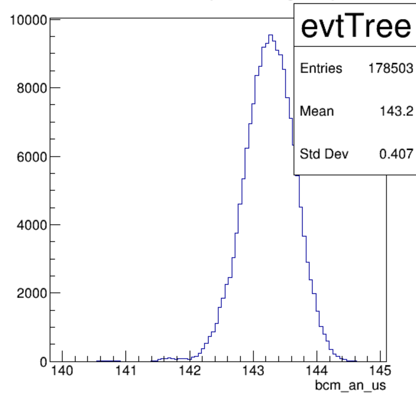
bcm_an_us {ErrorFlag==0}
