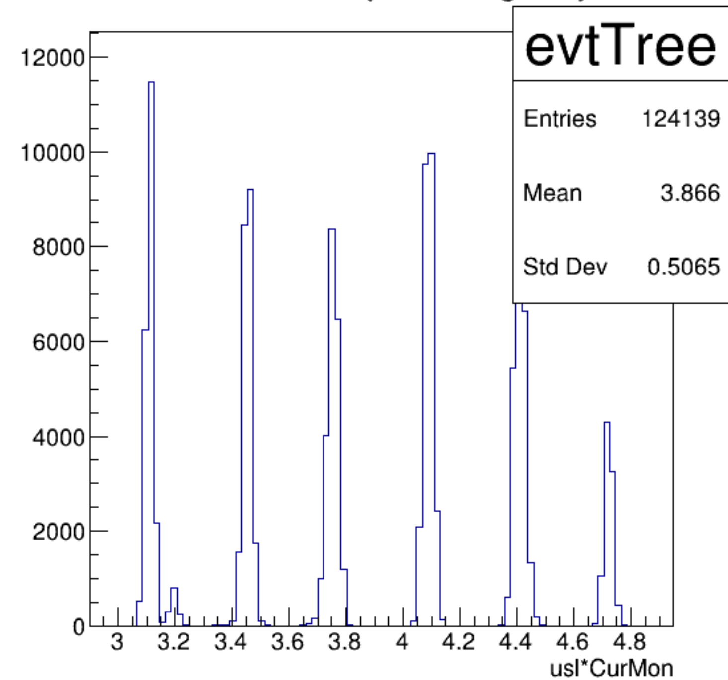
usl*CurMon {ErrorFlag==0}
