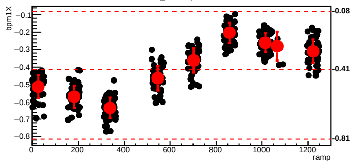
bmod_trim1,cyc=5862
