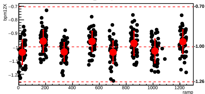
bmod_trim2,cyc=5862
