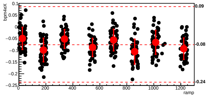
bmod_trim2,cyc=5862
