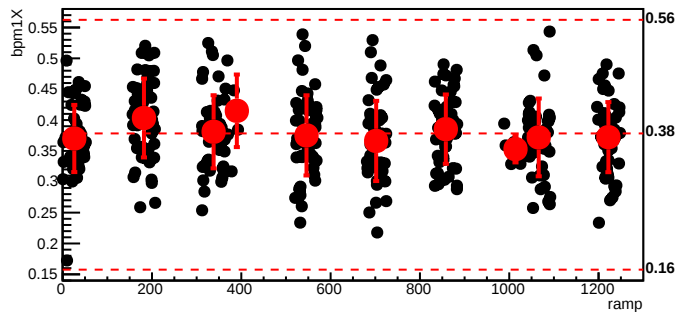
bmod_trim2,cyc=5955
