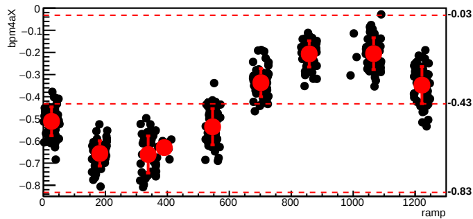
bmod_trim1,cyc=5955
