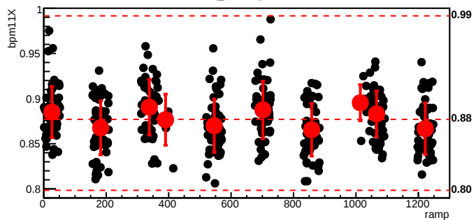
bmod_trim2,cyc=5955
