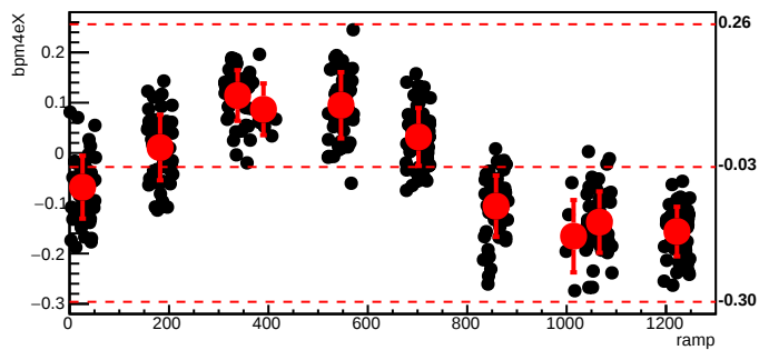
bmod_trim5,cyc=5955
