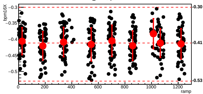
bmod_trim4,cyc=5955
