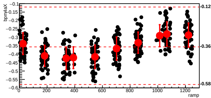
bmod_trim3,cyc=5955
