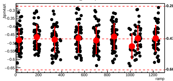
bmod_trim4,cyc=5955
