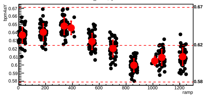
bmod_trim6,cyc=5955
