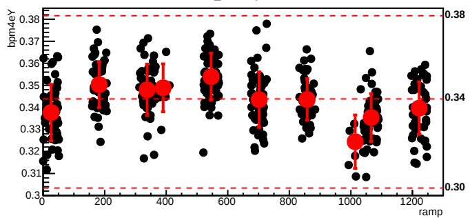
bmod_trim3,cyc=5955
