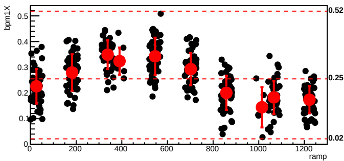
bmod_trim5,cyc=5955
