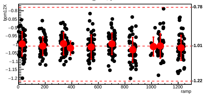
bmod_trim6,cyc=5955
