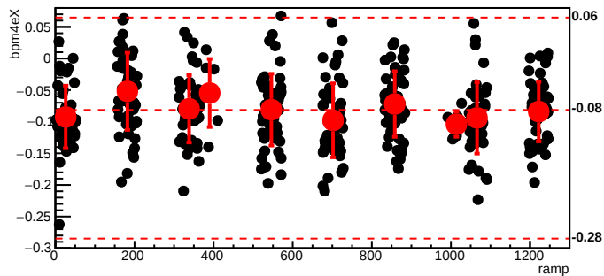
bmod_trim2,cyc=5955
