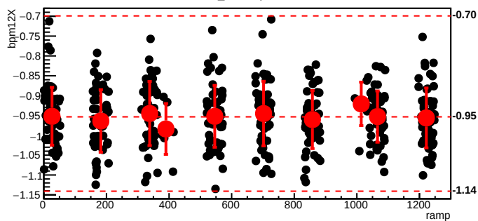
bmod_trim2,cyc=5955
