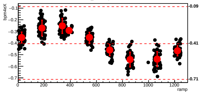
bmod_trim7,cyc=5957
