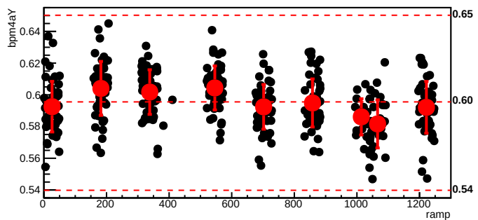
bmod_trim3,cyc=5977
