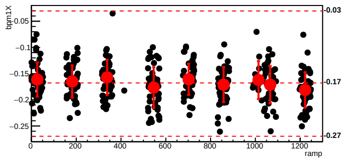
bmod_trim2,cyc=5977
