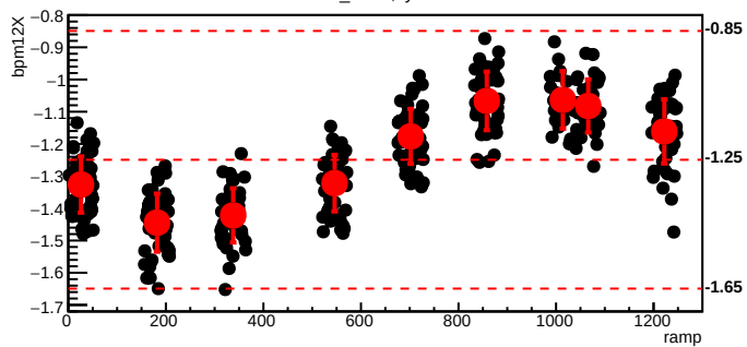
bmod_trim7,cyc=5977
