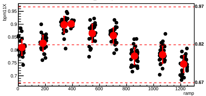
bmod_trim5,cyc=5995
