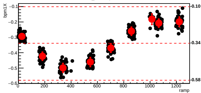
bmod_trim3,cyc=5995
