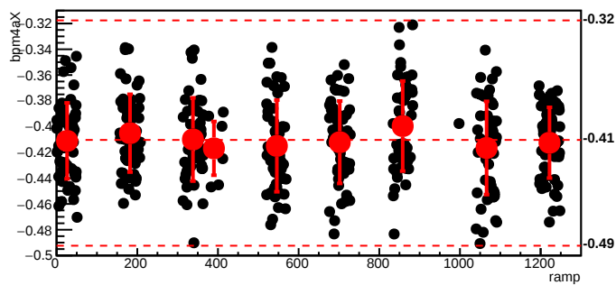
bmod_trim4,cyc=5995
