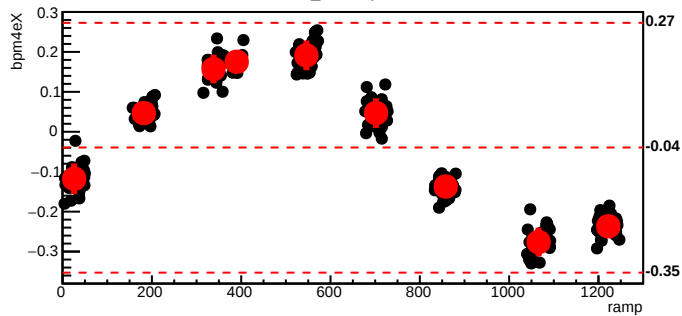
bmod_trim5,cyc=5995
