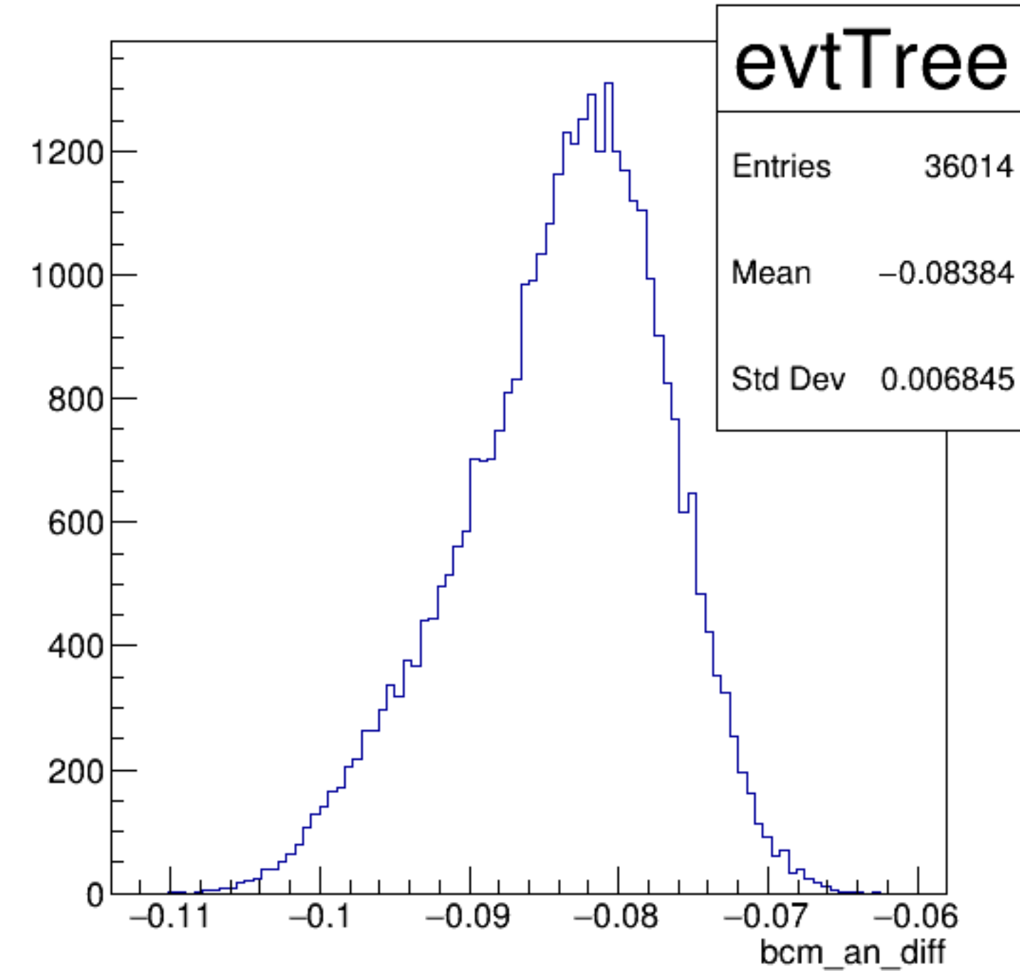
bcm_an_diff {ErrorFlag==0}
