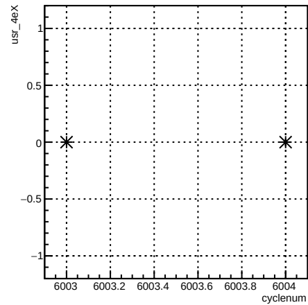
run:cyclenum {run == 6334}
