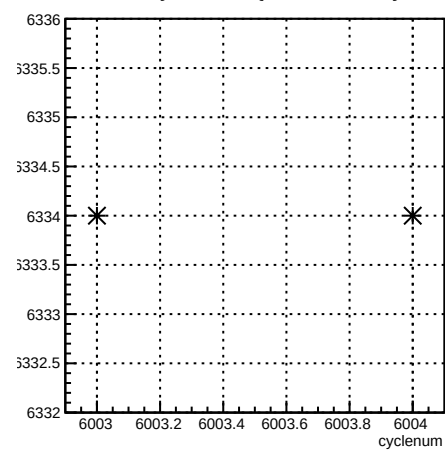
run:cyclenum {run == 6334}
