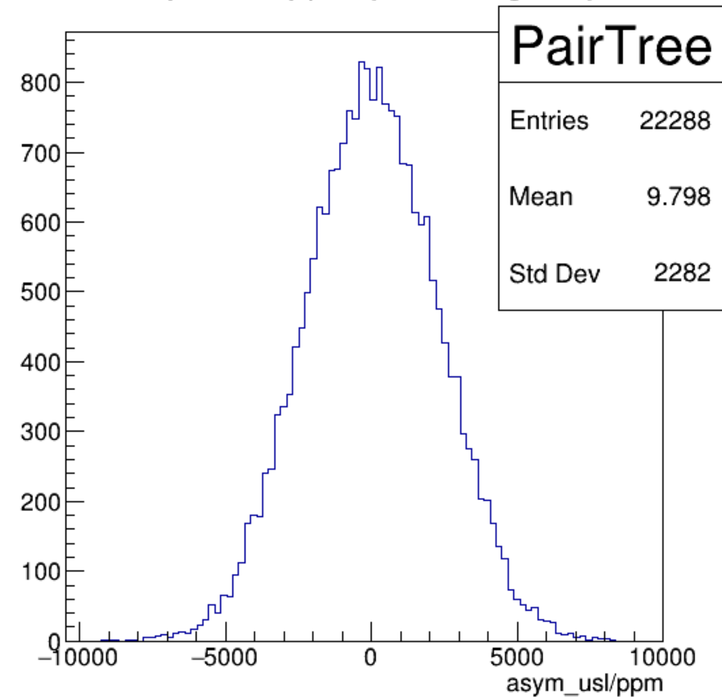
asym_usl/ppm {ErrorFlag==0}
