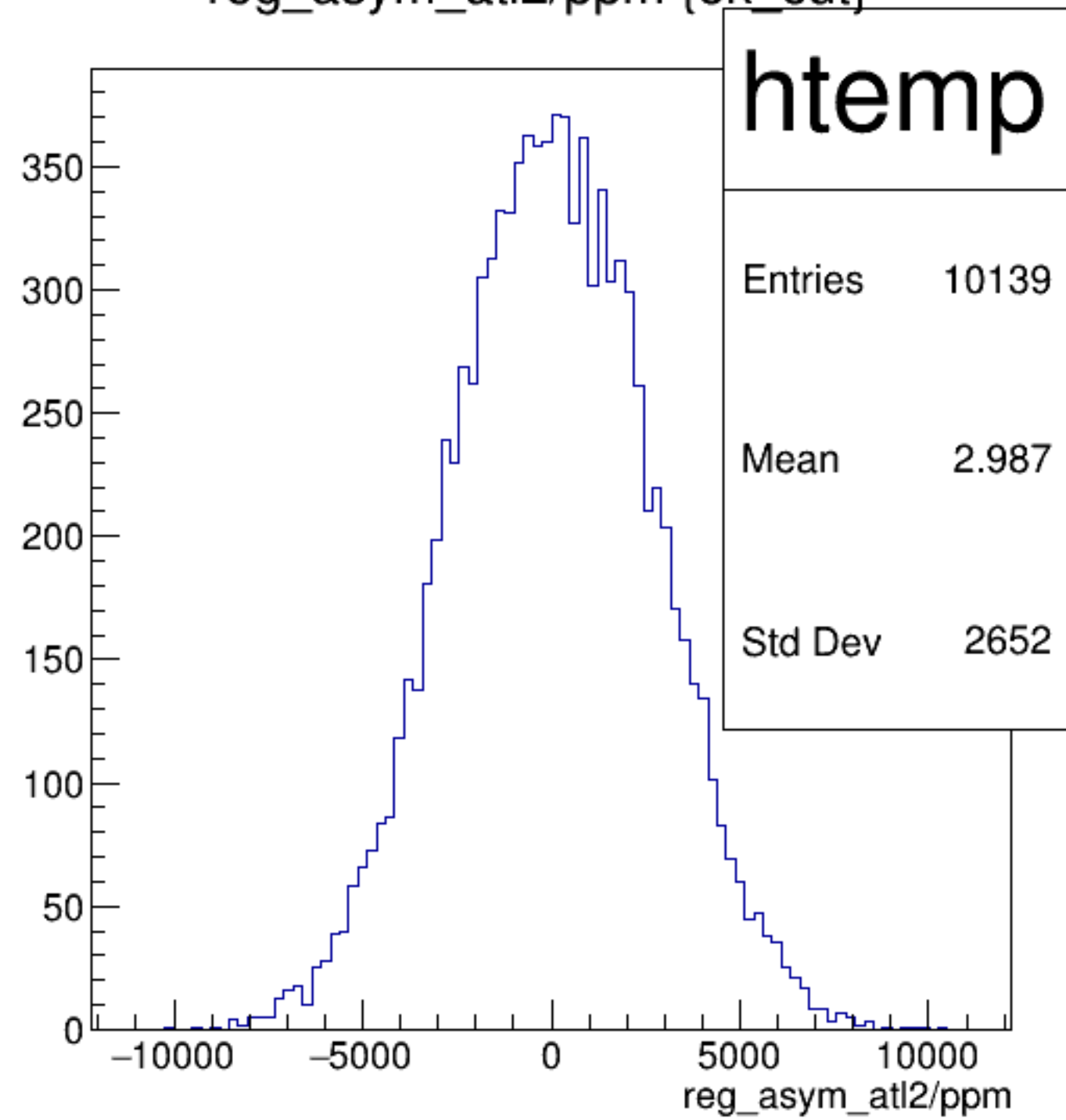
reg_asym_atl2/ppm {ok_cut}
