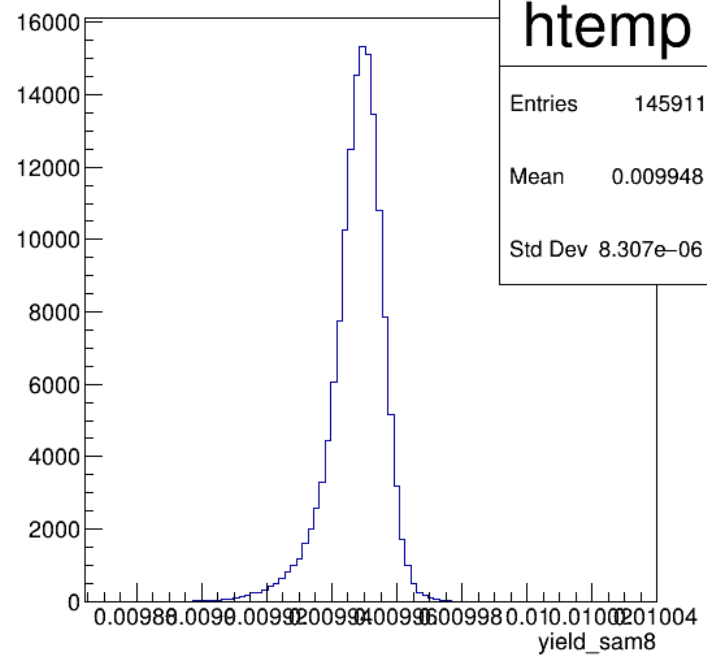
yield_sam8 {ErrorFlag==0}
