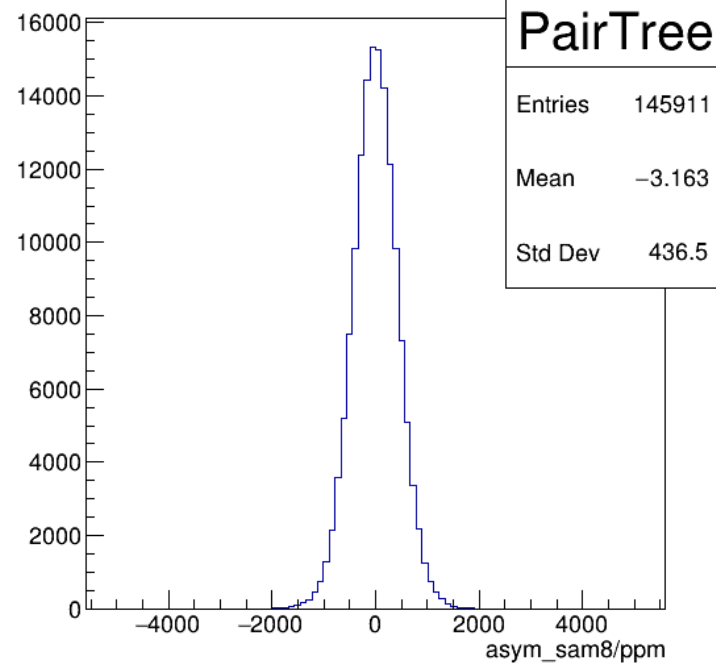
asym_sam8/ppm {ErrorFlag==0}
