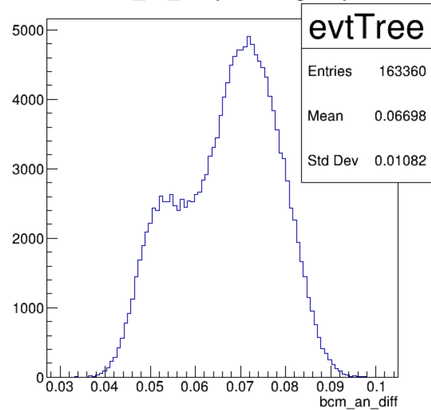
bcm_an_diff {ErrorFlag==0}
